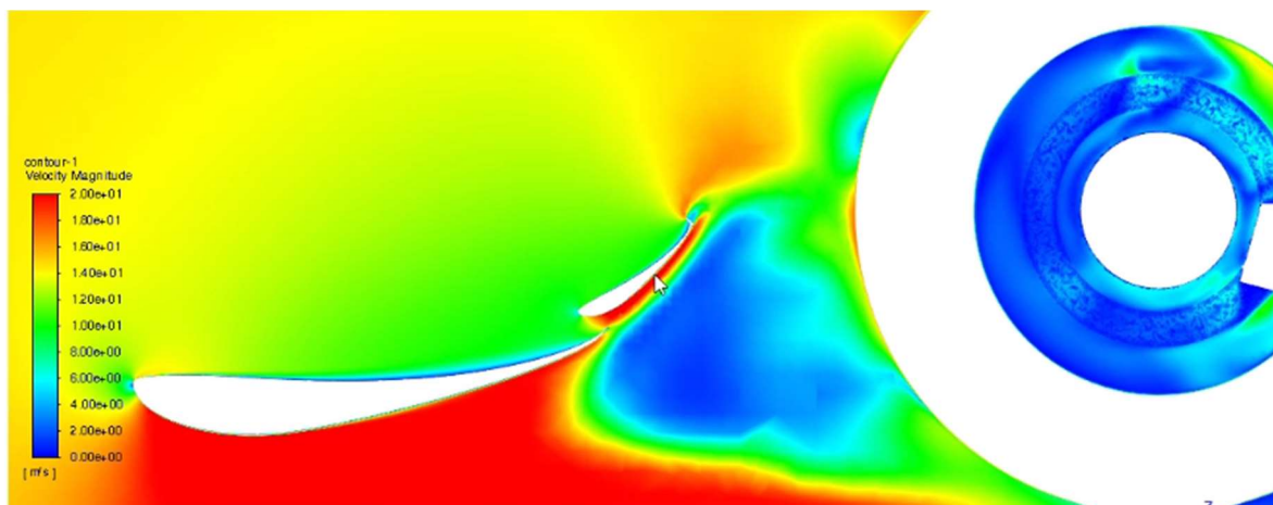
Obrázek č. 21 – Rychlost proudění okolo předního křídla v oblasti před kolem [autor práce]
