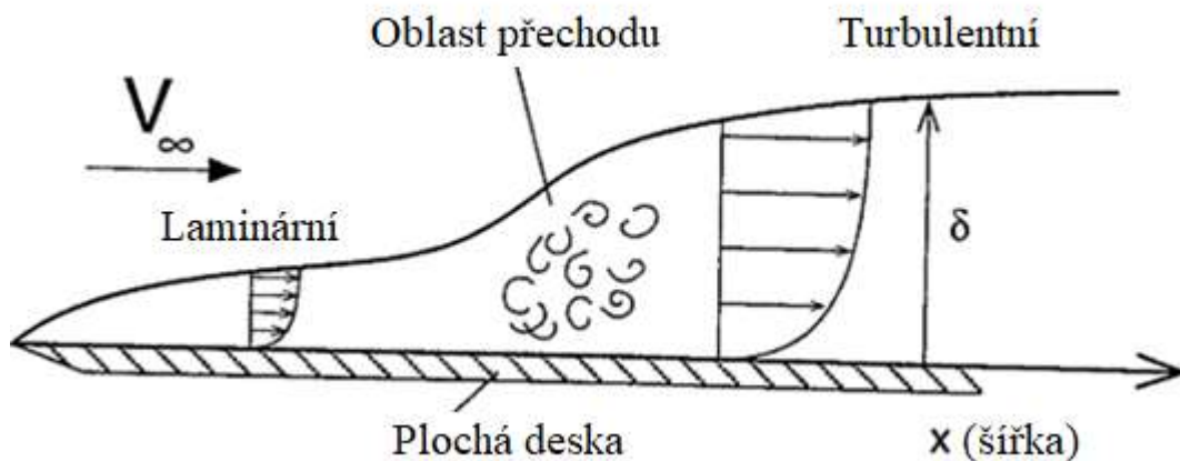
Obrázek č. 6 – Mezní vrstva podél ploché desky [12]
