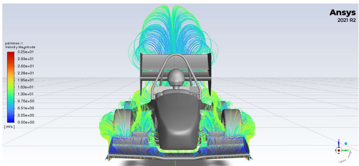
Obrázek č. 26 – Proudnicе vycházející z předního křídla [autor práce]
