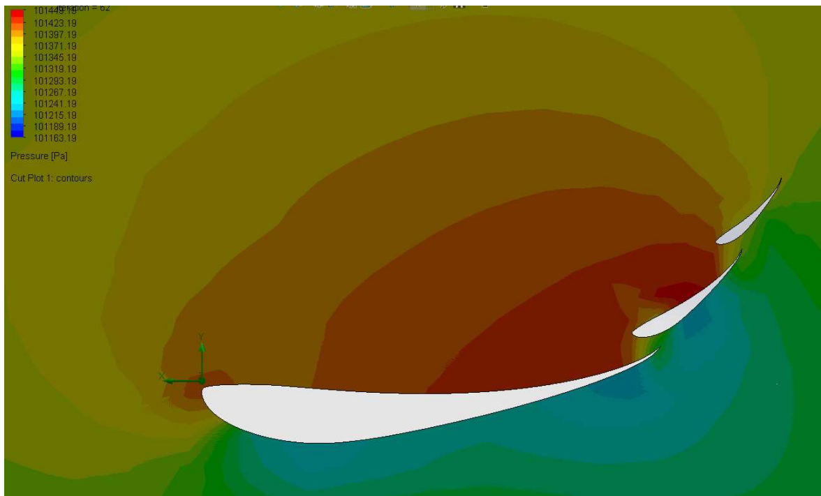
Obrázek č. 22 – Znáznornění rozložení tlaku okolo druhé varianty klapky [autor práce]
