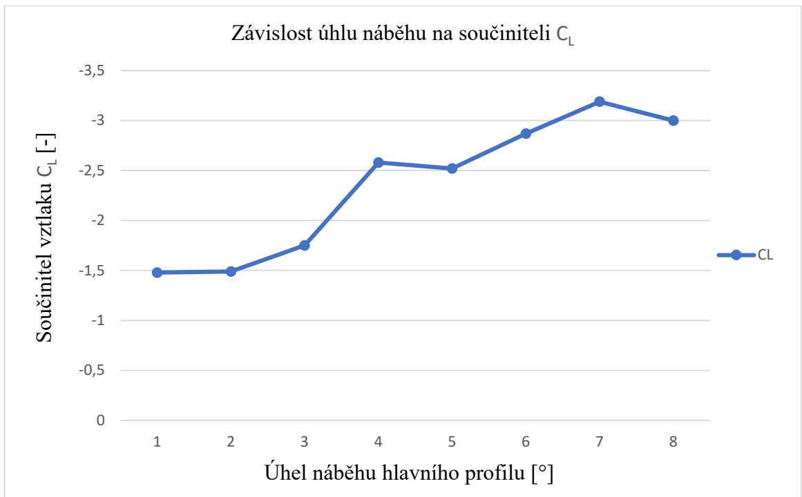
Obrázek č. 17 – Závislost úhlu náběhu na součiniteli vztlaku [autor práce]
