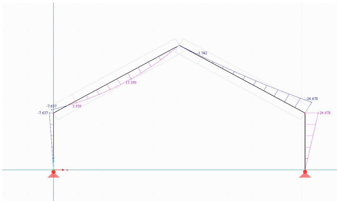
Obr.: Průběh ohybových momentů - kombinace zatížení KZ185
