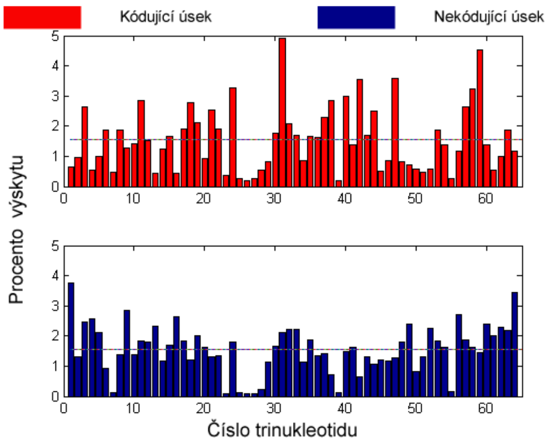
Obr. 21: Průměrný výskyt trinukleotidů v jednotlivých úsecích
