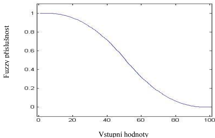
Obr. 1: Graf Z-funkce
