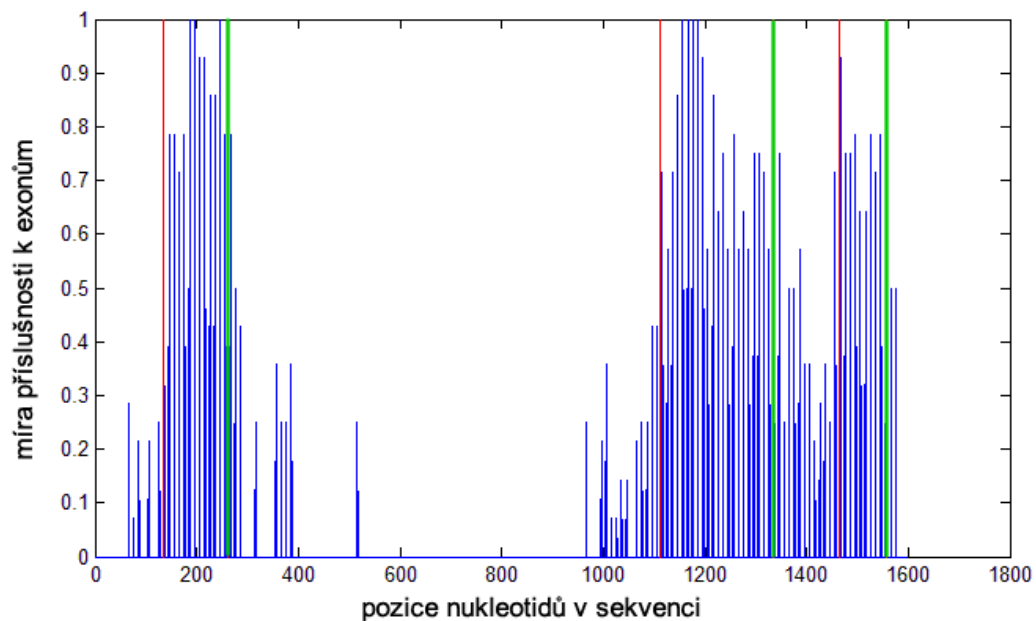
Obr. 31: Minimální příslušnost (okno délky 50 se skokem po 10)
