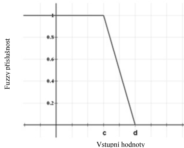
Obr. 4: Graf Rfunkce
