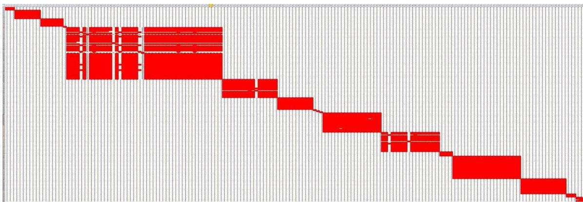
Obr. 39: Červené vyznačení FMF=1 na celém souboru 180 sekvencí (Euklidovská vzdálenost)
