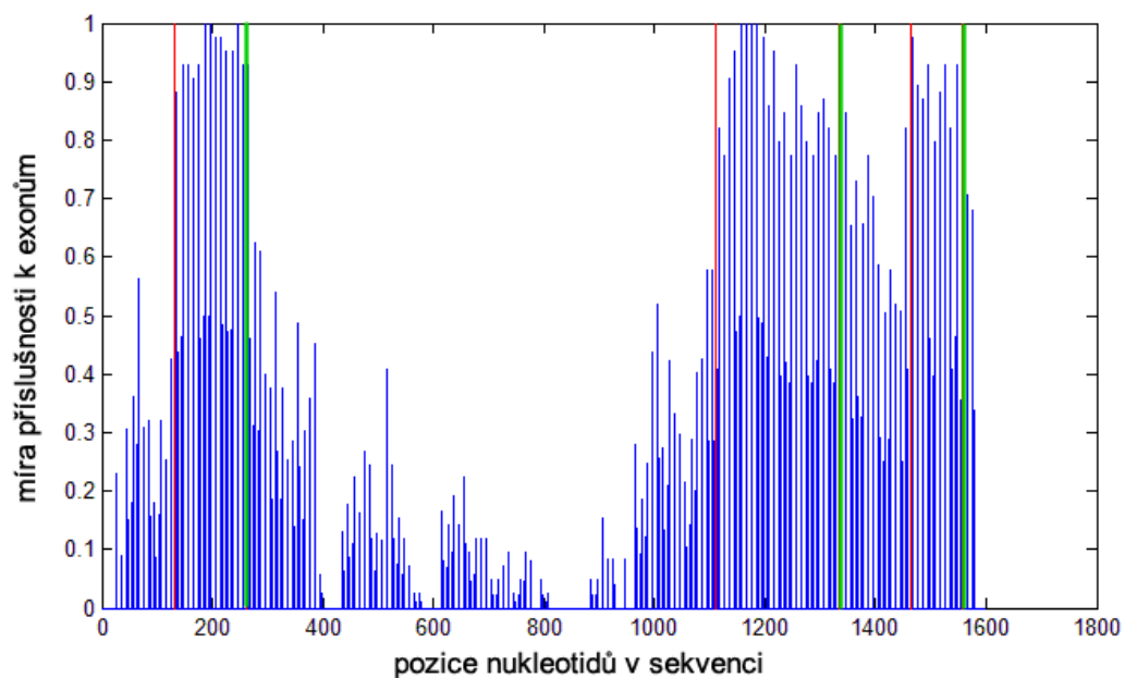
Obr. 30: Průměr příslušností (okno délky 50 se skokem po 10)
