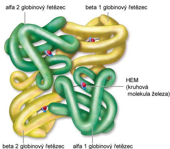
Obr. 17: Molekulová struktura hemoglobinu [21]
