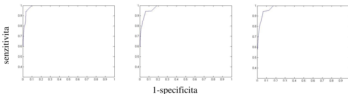
Obr. 41: ROC křivky pro FMF-D15, FMF-D30 a FMF-JC
