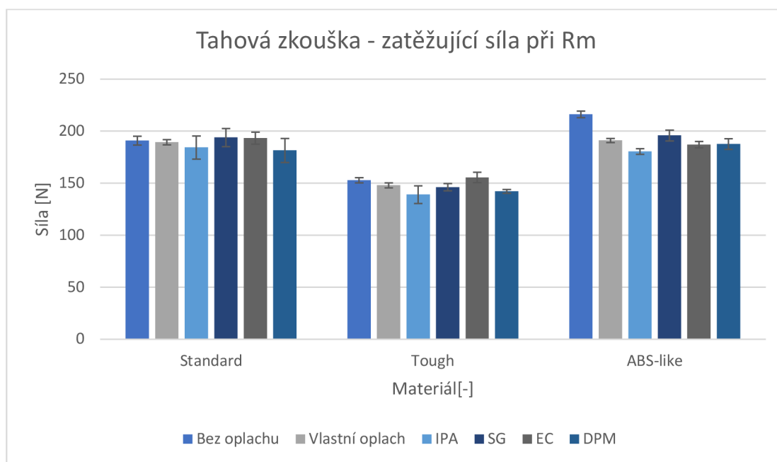
Obr. 78 Výsledky zatěžujících sil při Rm v průběhu tahové zkoušky testovaných materiálů.
