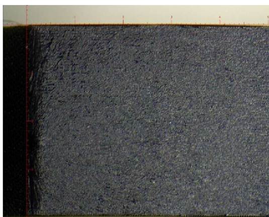
Obr. 75 Lom materiálu Tough po 10 min oplachu DPM.
