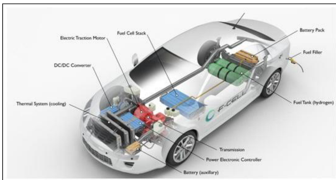
Obr. 1: Konstrukce vozidla FCEV [14]
