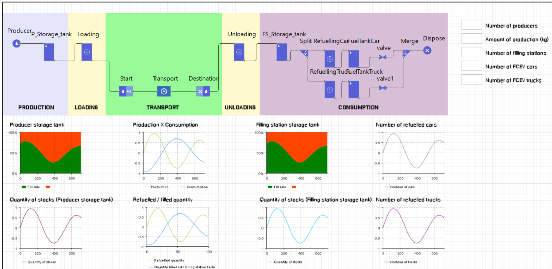
Příloha. 1: Model pro verifikaci výsledků [vlastní zpracování s využitím [46]]
