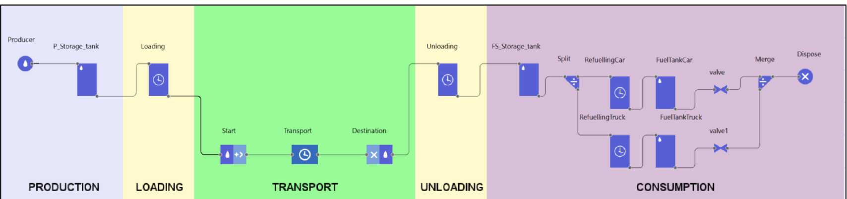
Obr. 26 Model pro verifikaci výsledků – proces výroby, distribuce a spotřeby vodíku [vlastní zpracování s využitím [46]]
