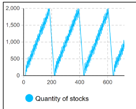
Obr. 28: Stav zásobníků PS v kg [vlastní zpracování s využitím [46]]
