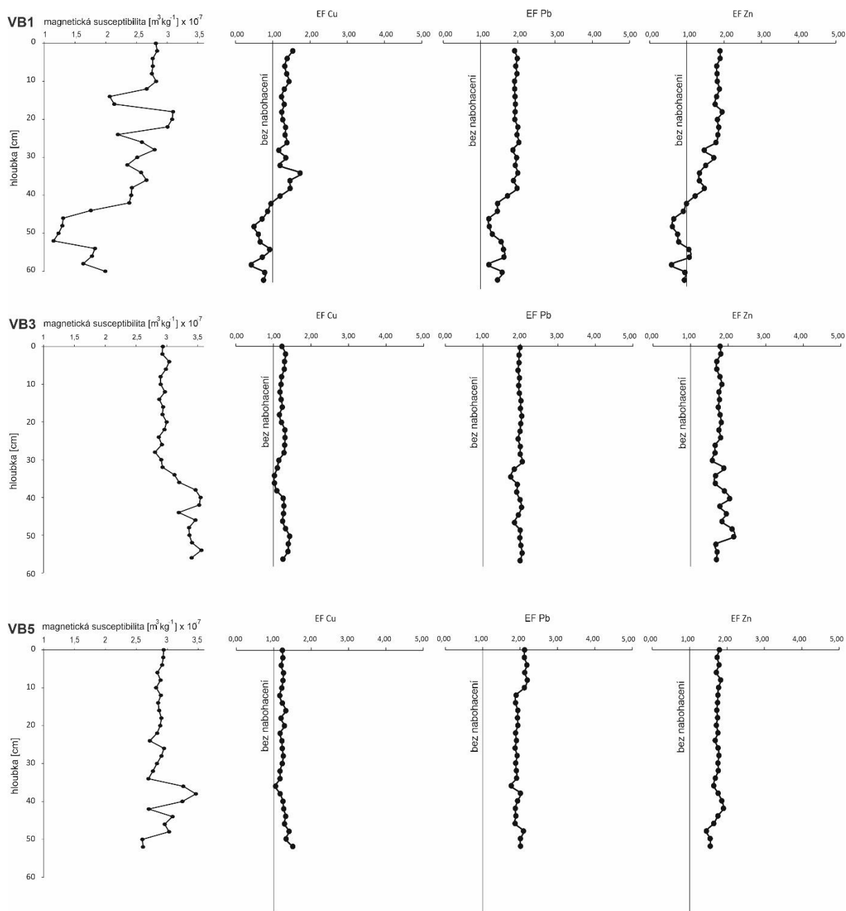
Obrázek 32: Znázornění korelace křivek magnetické susceptibilita a EF těžkých kovů v jednotlivých jádrech VB1, VB3 a VB5.
