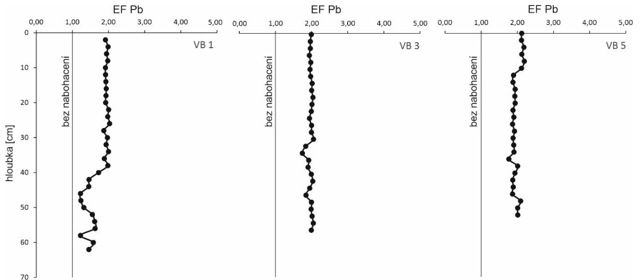
Obrázek 23: Grafické znázornění závislosti faktoru nabohacení Pb na hloubce pro jádra VB1, VB3 a VB5.
