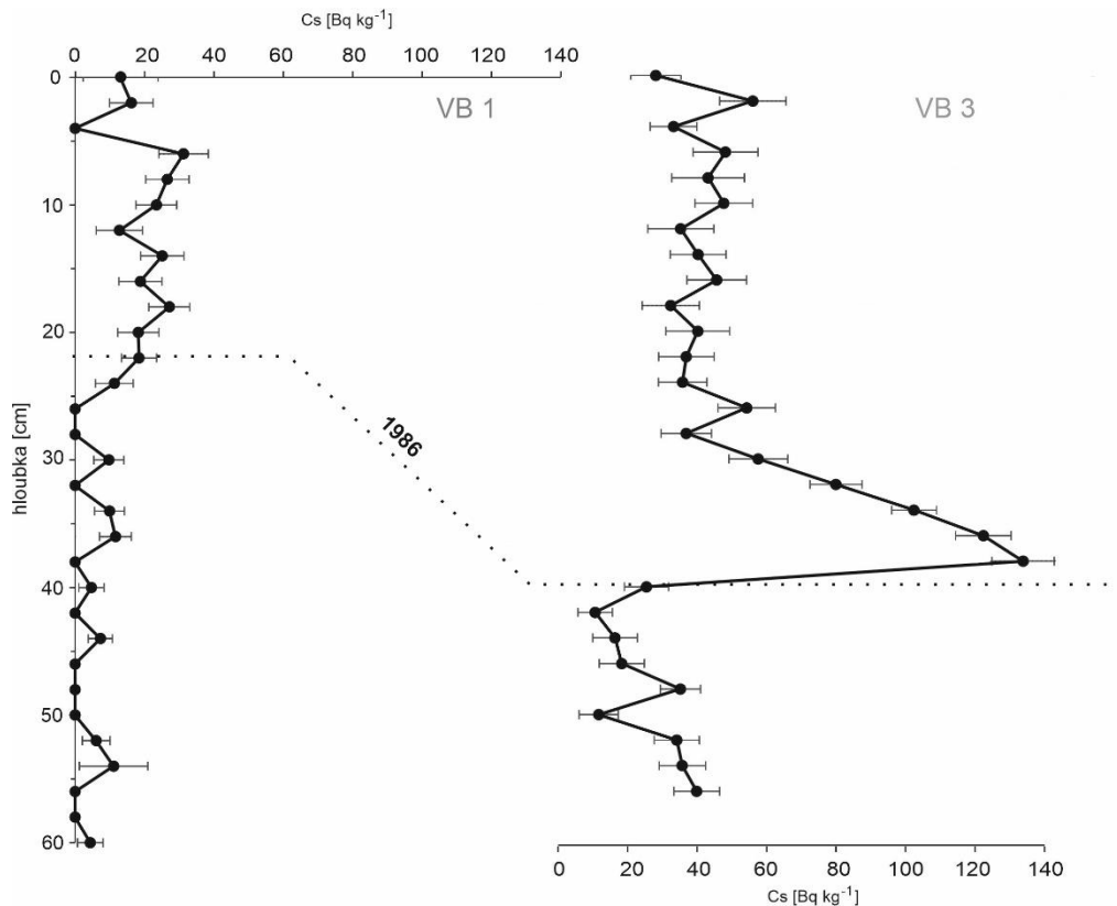
Obrázek 15: Grafické znázornění závislosti hmotnostní aktivity radioizotopu ^{137}\text{Cs} na hloubce u jader VB1 a VB3.
