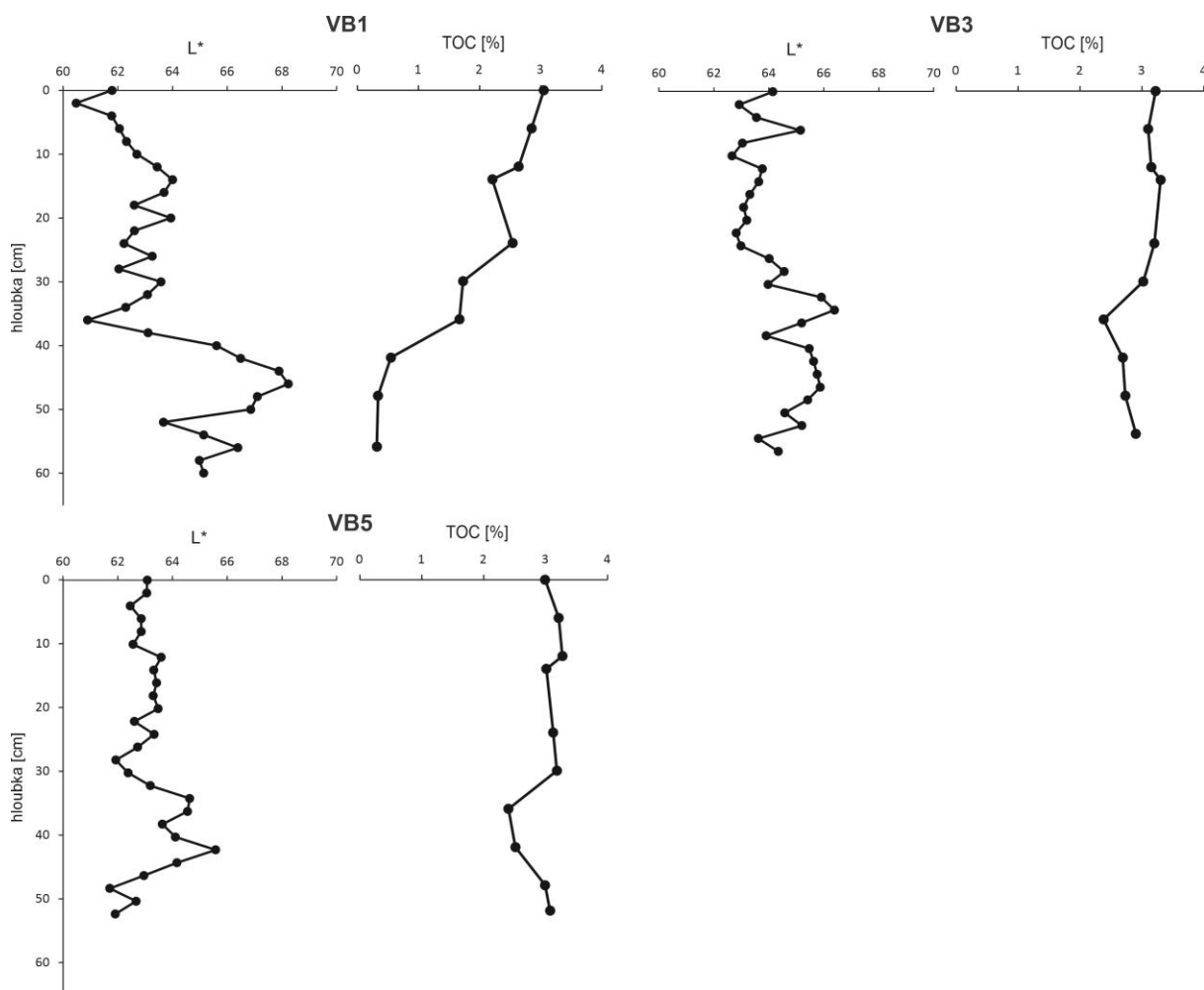
Obrázek 34: Znárodnění korelace křivek parametru L^* a obsahu TOC v jednotlivých jádrech VB1, VB3 a VB5.
