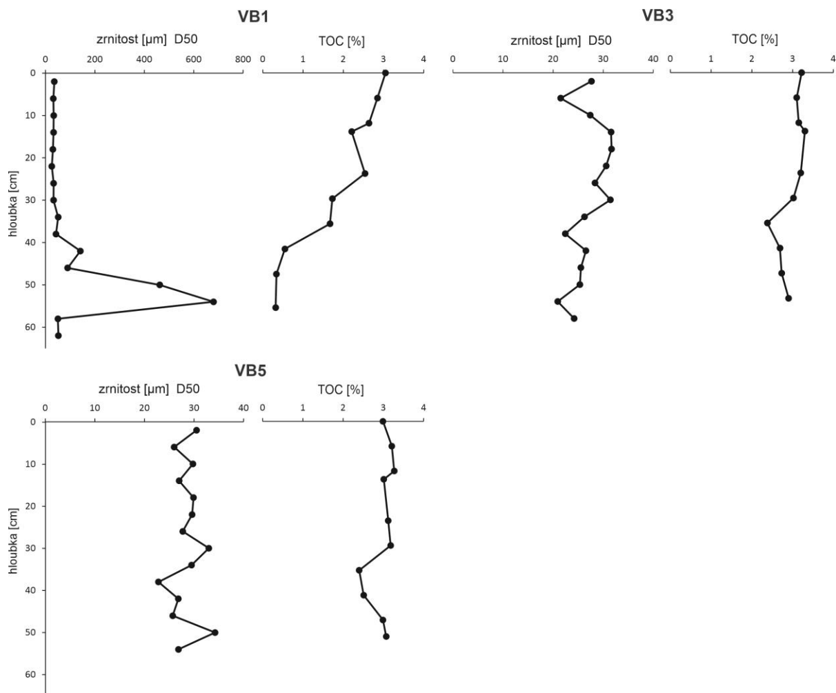
Obrázek 30: Znáornění korelace křivek střední velikosti zrna a obsahu TOC v jednotlivých jádrech VB1, VB3 a VB5.
