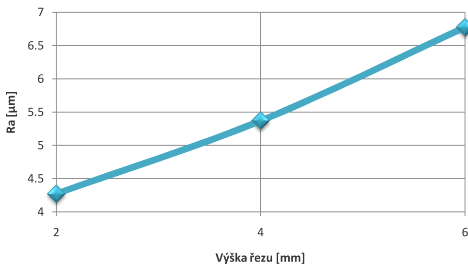
Obr. 5.6 Vliv výšky řezu na hodnotu R_a .
