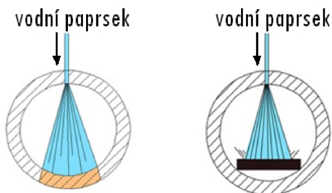
Obr. 1.11 Řezání dutého profilu [17].
