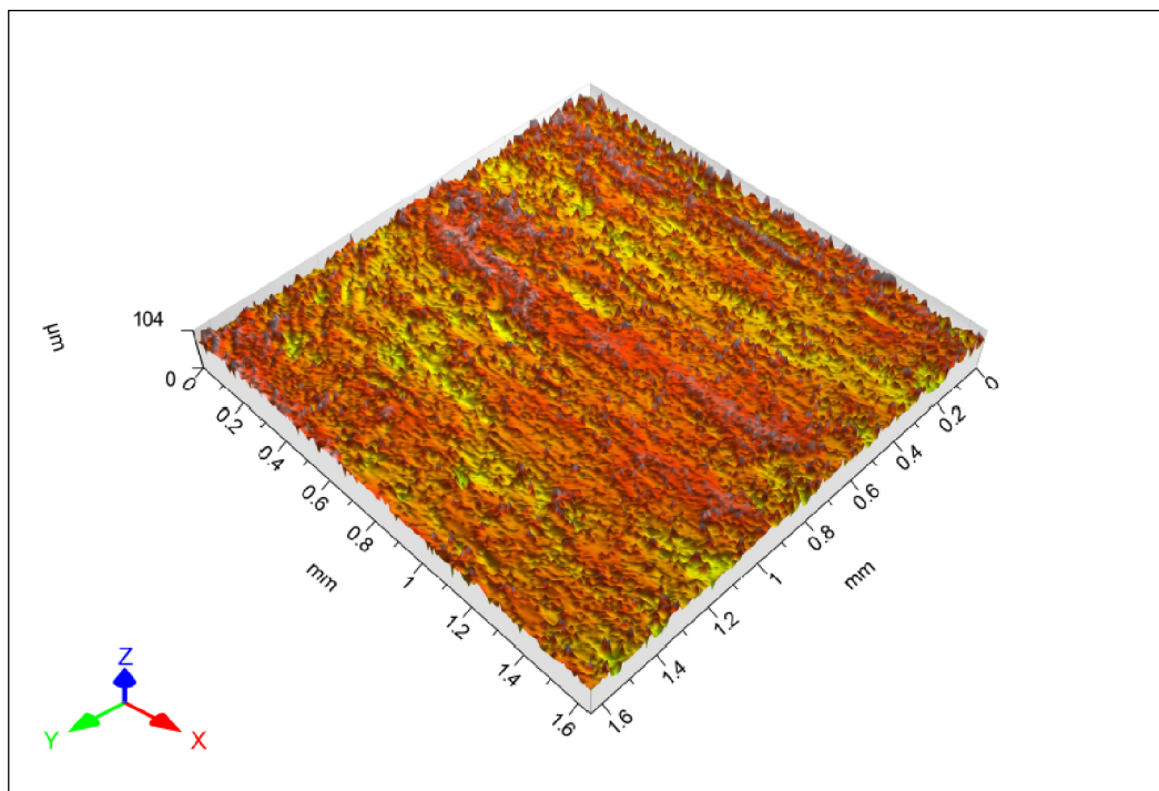
Obr. 5.4 Nasnímaná textura povrchu vzorku č. 1.1.
