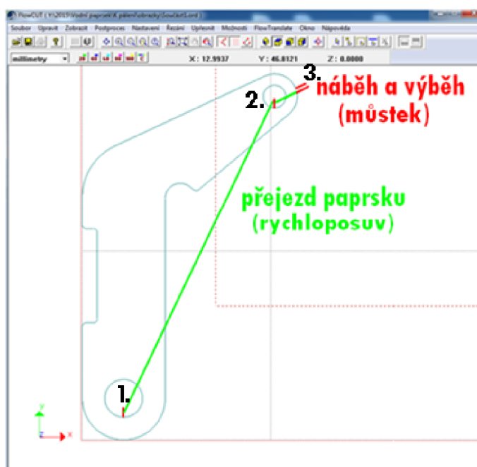
Obr. 4.7 Náběhy a výběhy pro řeznou dráhu.
