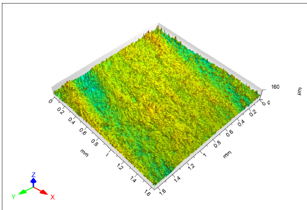
Obr. 5.5 Nasnímaná textura povrchu vzorku č. 3.3.
