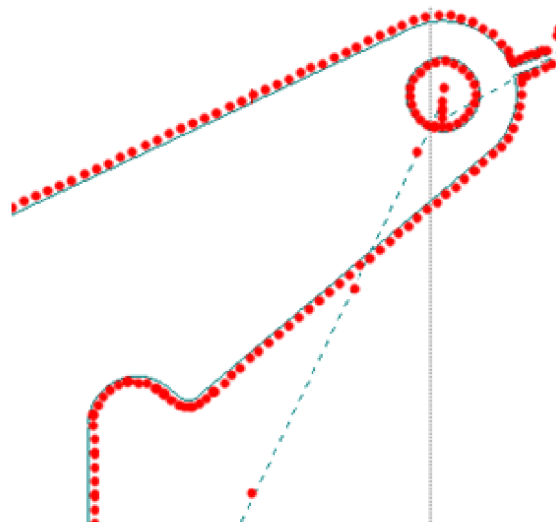
Obr. 4.9 Detail řezné dráhy.
