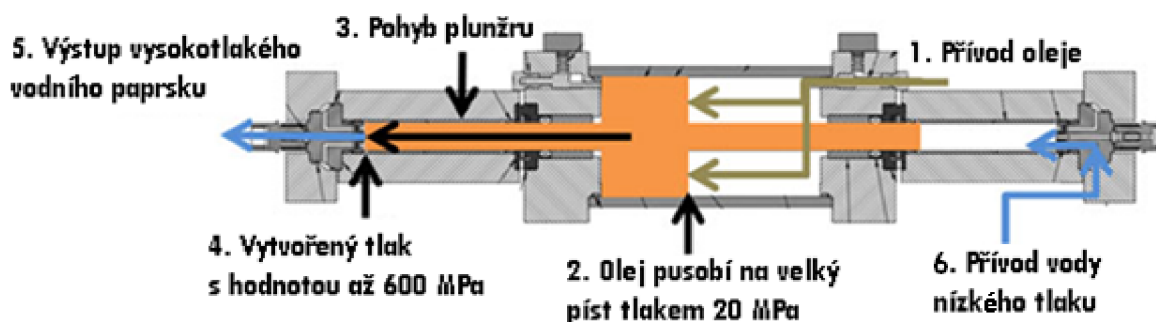
Obr. 2.1 Princip multiplikátoru [11].
