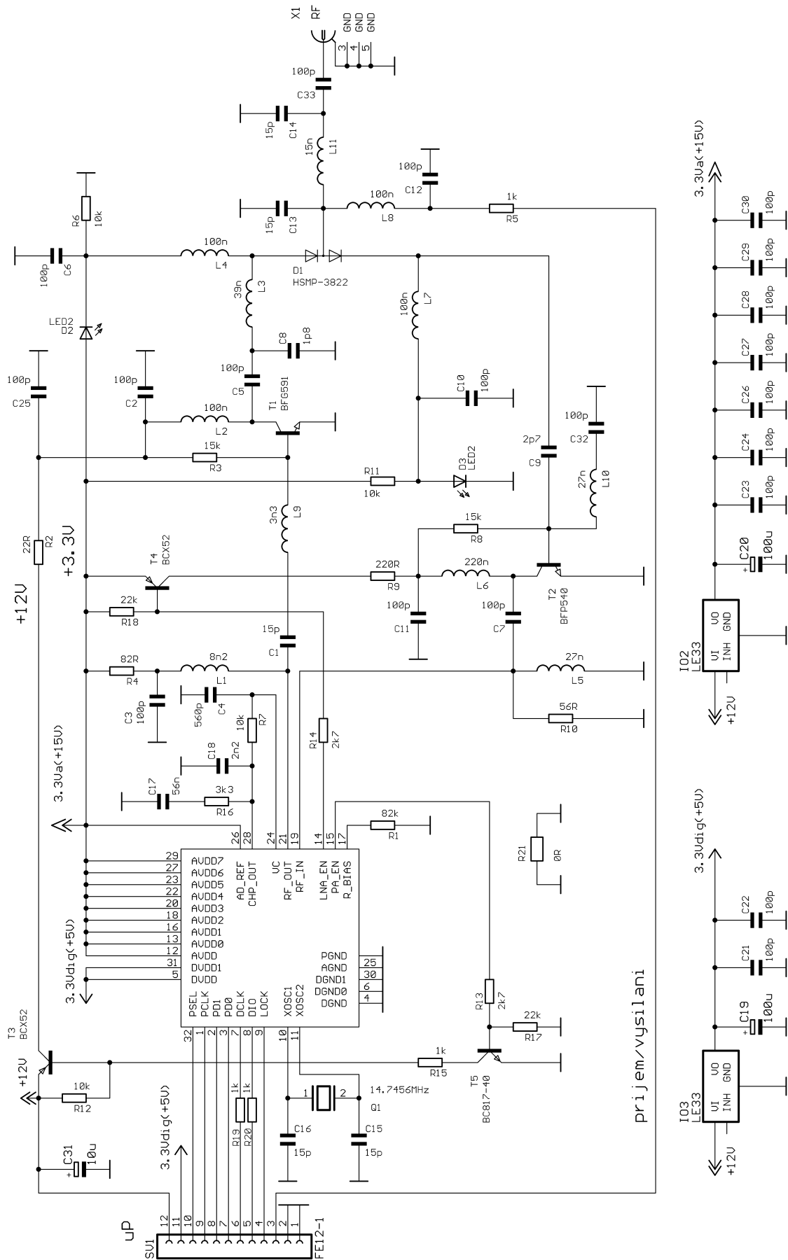
Obr. 22 Schéma zapojení modulu
