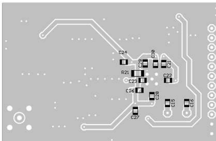
Obr. 30 Osazení modulu ze strany spojů
