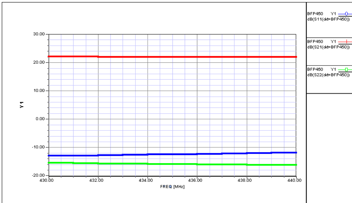
Obr. 18 Přizpůsobení LNA pro pracovní kmitočty
