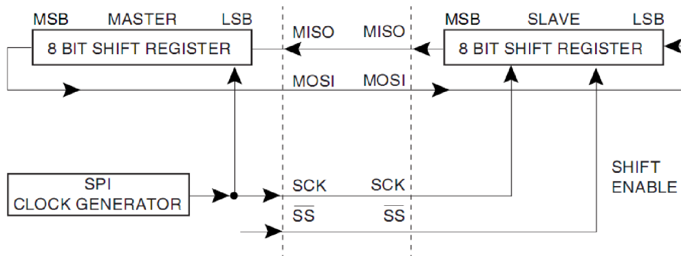
Obr. 24 Princip SPI
