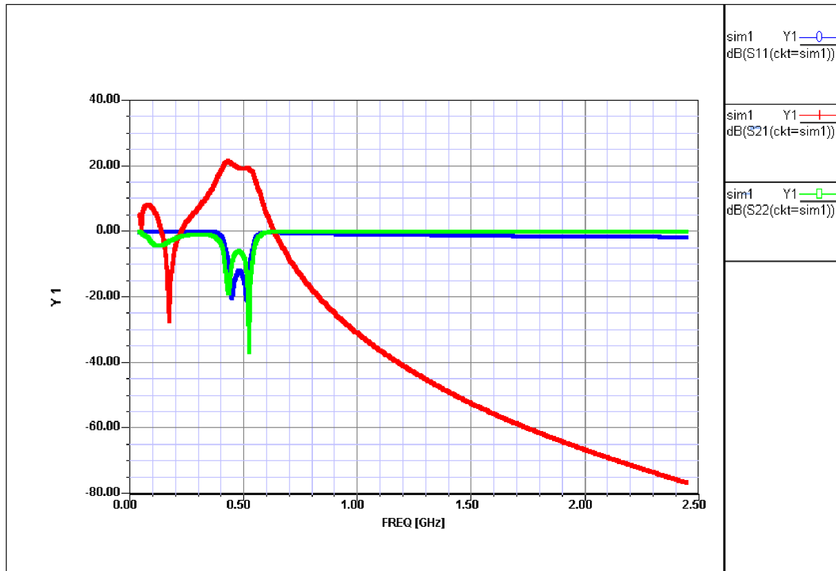
Obr. 16 Přizpůsobení PA pro 0 - 2,5 GHz
