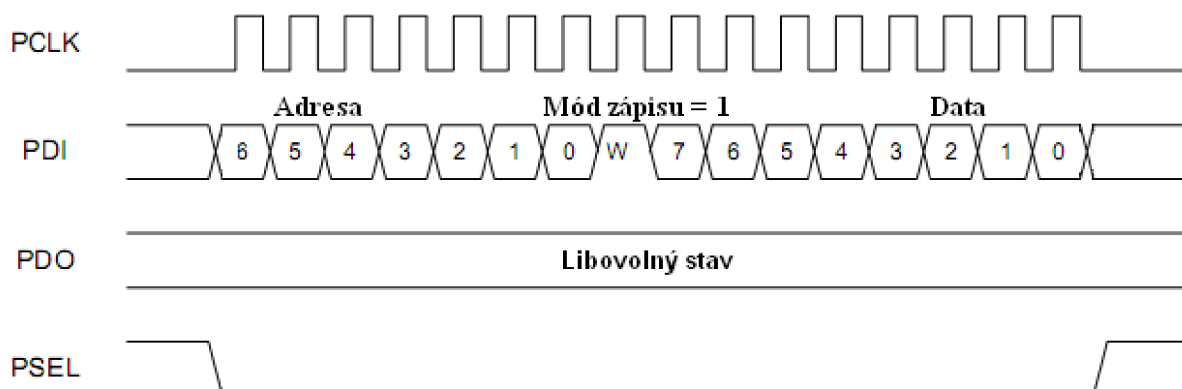
Obr. 7 Časování řídicího rozhraní, zápis do registru
