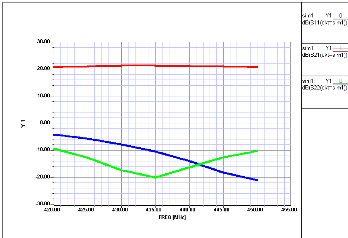
Obr. 15 Přizpůsobení PA pro pracovní kmitočty
