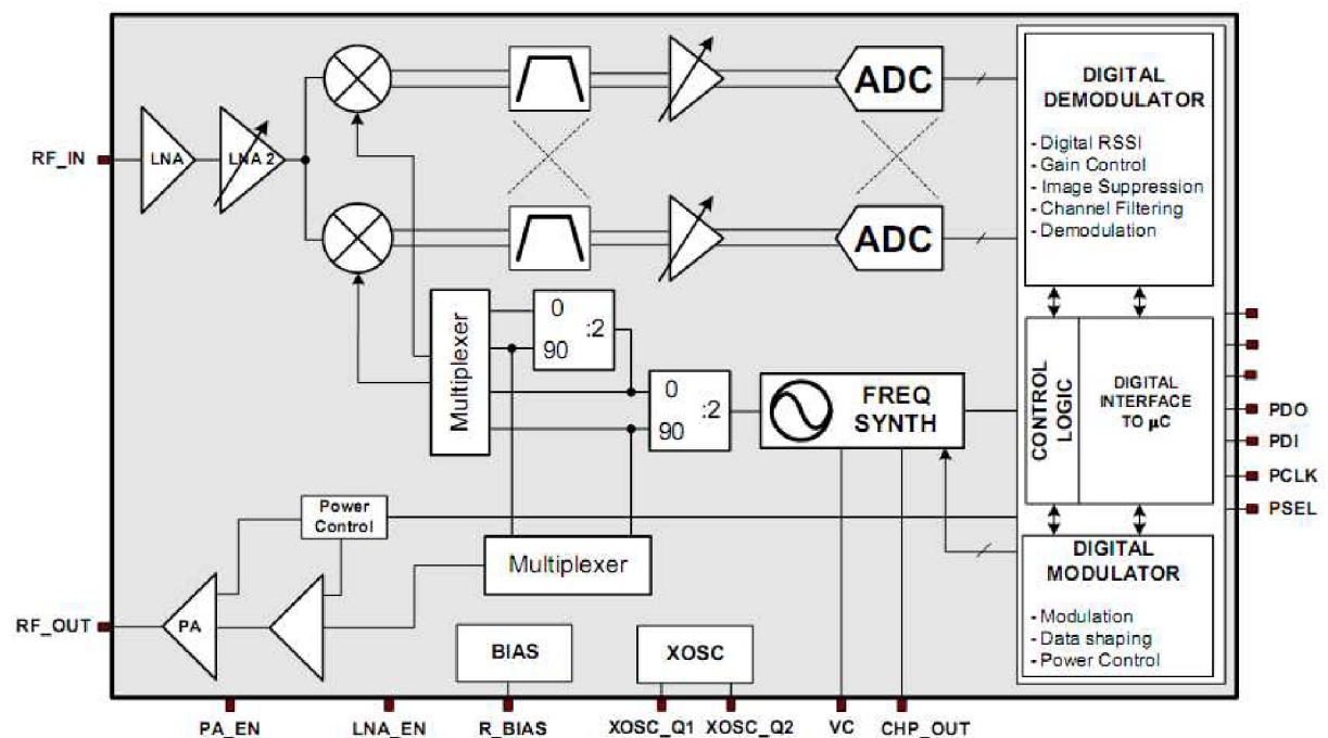
Obr. 3 Blokové schéma obvodu CC1020
