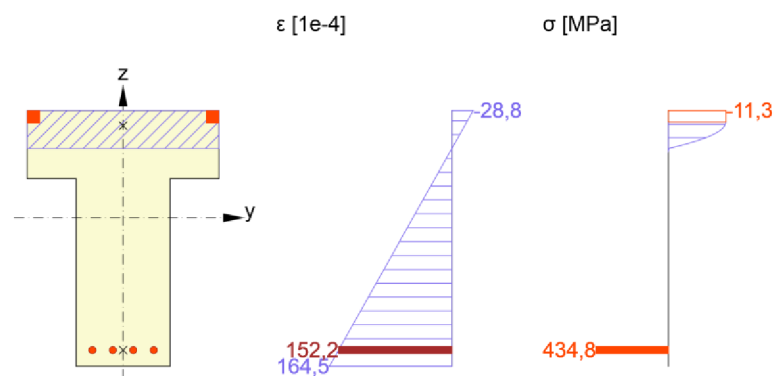
Obr. 2-8 Rozdělení přetvoření a napětí při ohybu u ŽB průřezu
