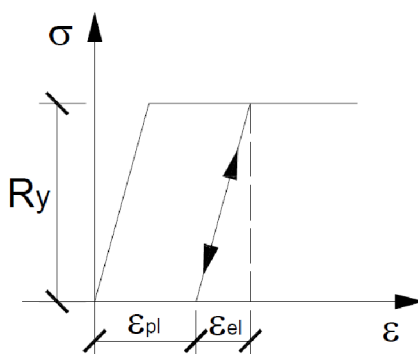
Obr. 2-5 Pracovní diagram pro ideálně pružně-plastický materiál
