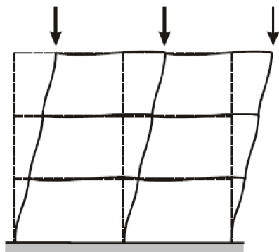
Obr. 2-12 P- \Delta efekt na konstrukci
