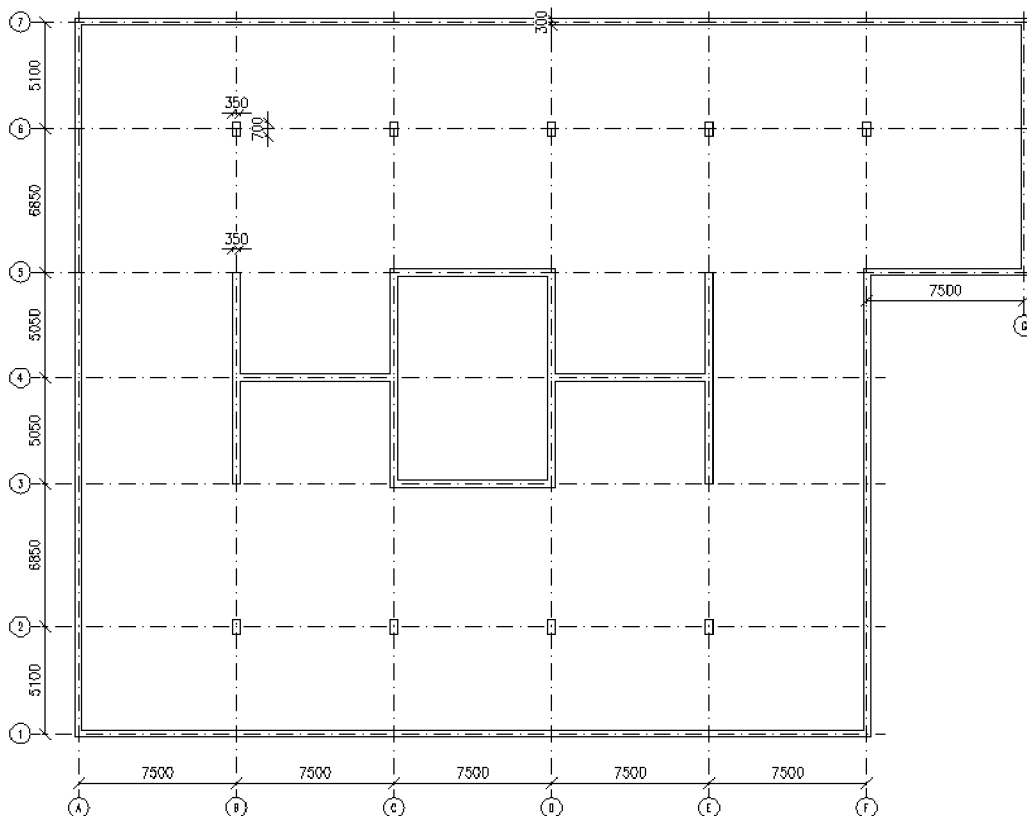
Obr. 3-5 Půdorys 1-3PP
