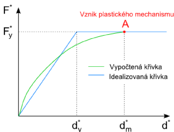
Obr. 2-13 Graf závislosti pružněplastické síly F^* na posunu d^*
