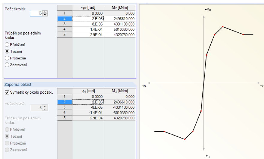
Obr. 3-39 Graf závislosti M - \varphi kolem osy Z (pro průřez reprezentativního patra) jen pro program RFEM
