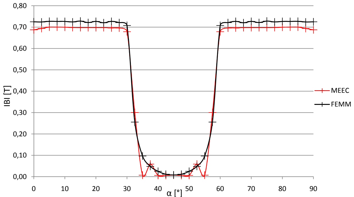
Obr. č. 25 |B| = f(\alpha) metódami MEEC a FEMM aplikovaním carterovho činiteľa
