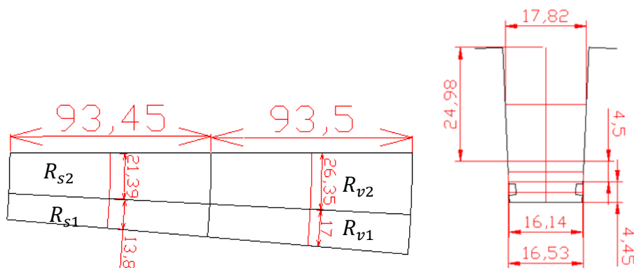
Obr. č. 21 a) Rozmery statorovej časti
