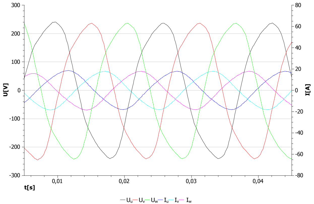
Obr. č. 50 Priebehy napätí a prúdov pri induktívnej záťaži \cos\varphi = 0,8 .
