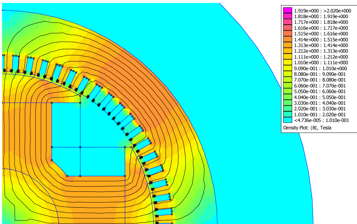
Obr. č. 12 Rozloženie magnetického toku pre 0-90°
