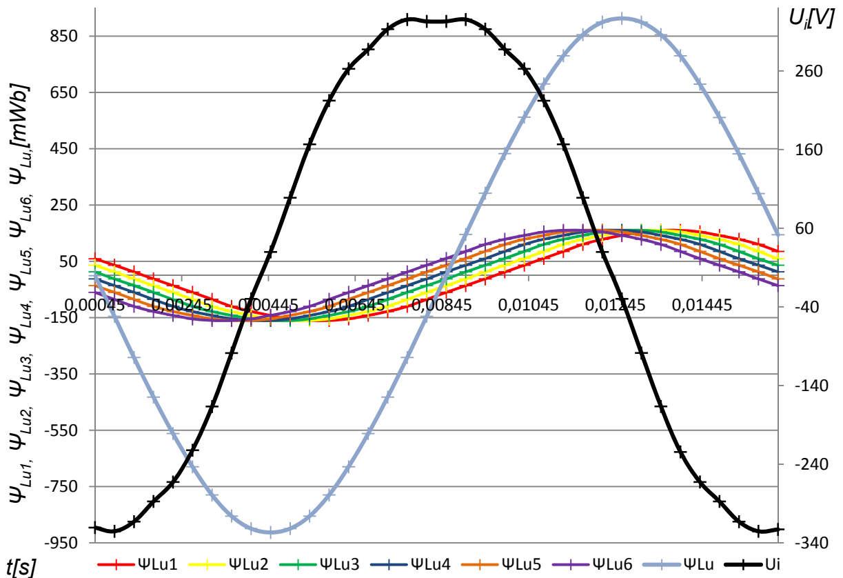
Obr. č. 28 Priebeh čiastkových magnetických tokov závitmi vinutia a ich súčet.
