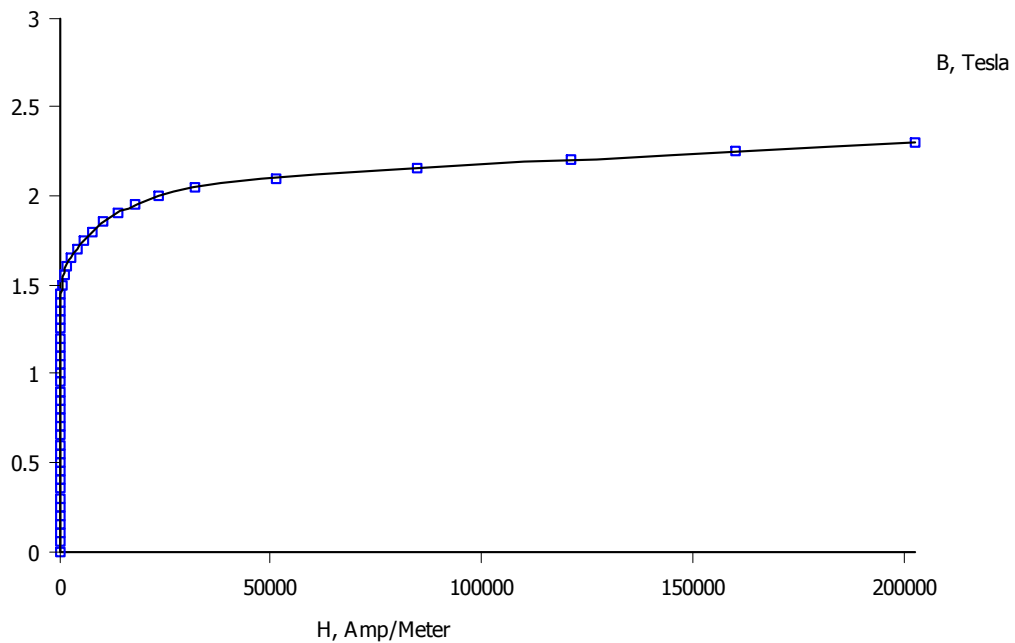
Obr. č. 45 Magnetizačná charakteristika použitého plechu
