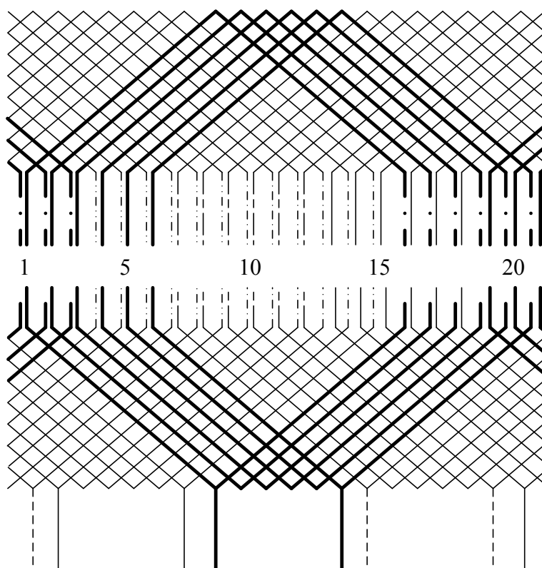
Obr. č. 9 Uloženie dvojrstvového vinutia
