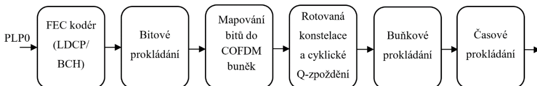
Obr. 2 Blokový diagram BICM (na základě [8])
