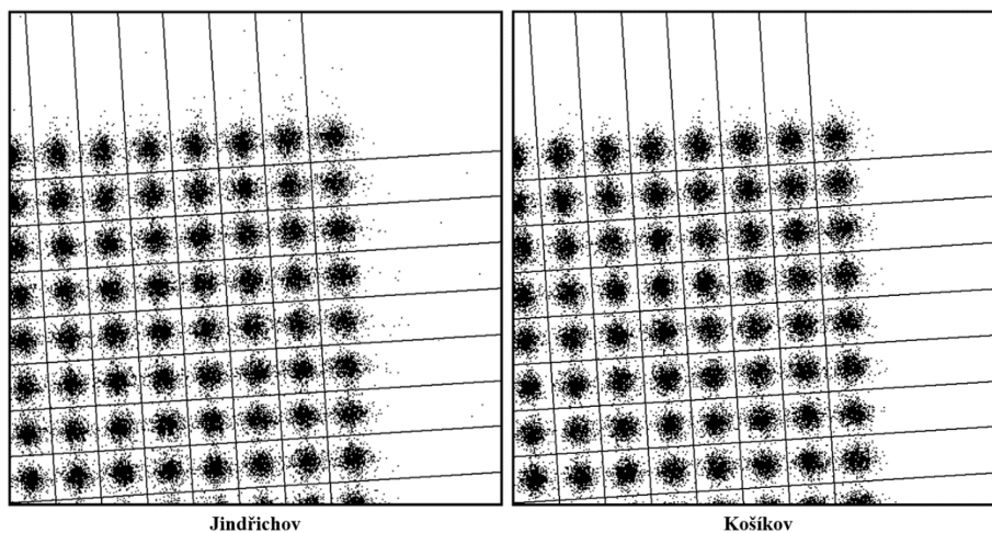
Obr. 52 Konstelační diagramy 256-QAM, první kvadrant, vysílač Brno-Kojál – třetí terénní měření
