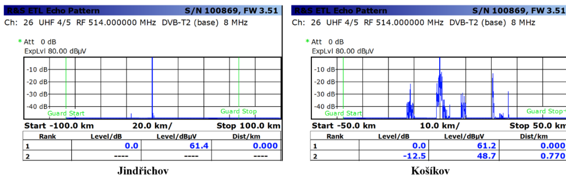
Obr. 53 Echo vybraných míst, vysílač Jihlava-Javořice – třetí terénní měření
