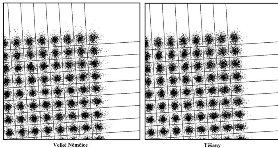
Obr. 44 Konstelační diagramy 256-QAM, první kvadrant, vysílač Brno-Kojál – druhé terénní měření
