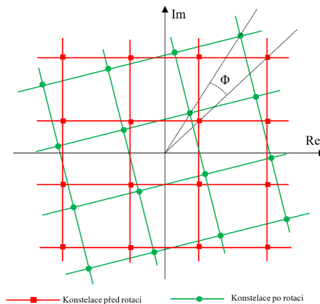
Obr. 3 Rotovaný konstelační diagram modulace 16-QAM (na základě [11])
