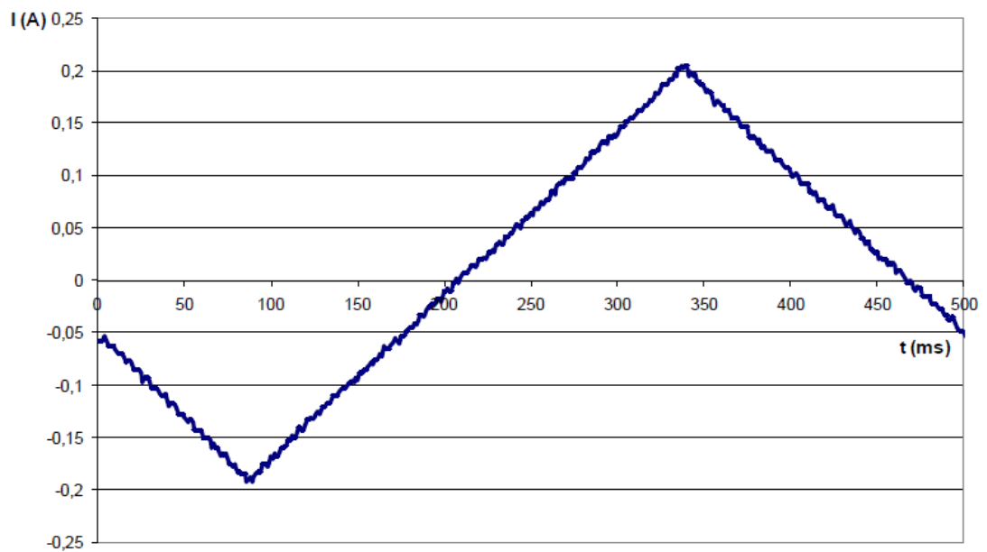
Obr. 7.11: Trojuholníkový signál
