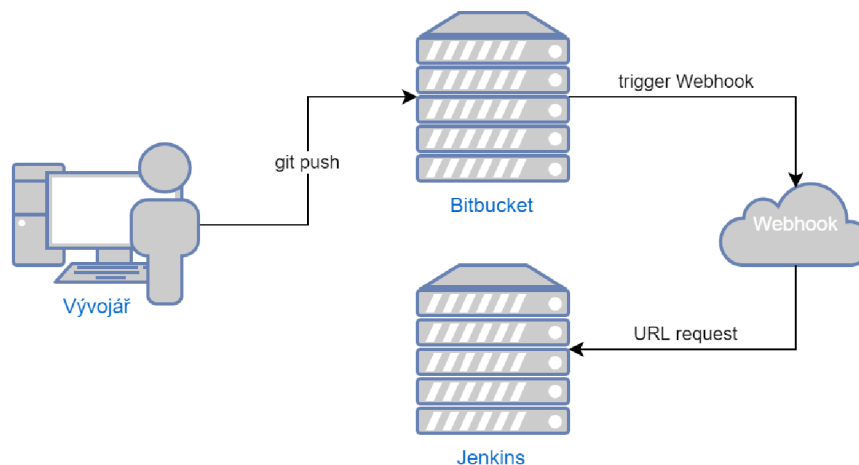
Obrázek 3.3: Bitbucket Webhook
