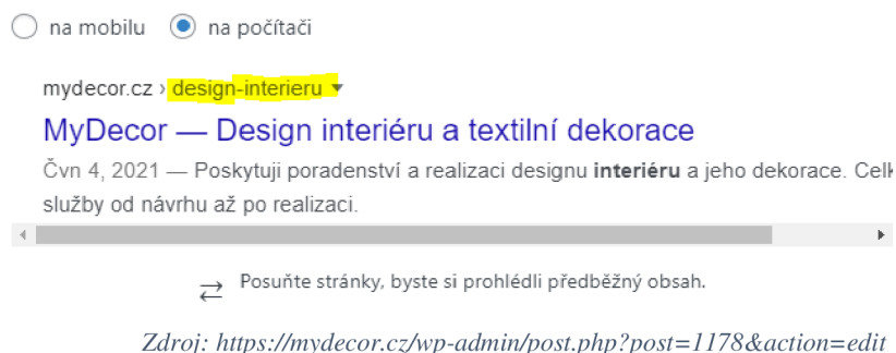
Obrázek 21 - slug
