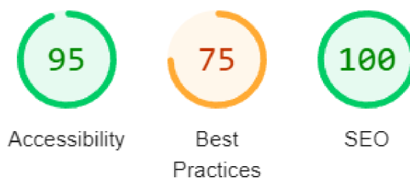
Obrázek 22 – skóre Lighthouse
