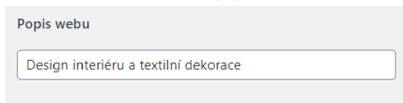
Obrázek 19 – popis webu
