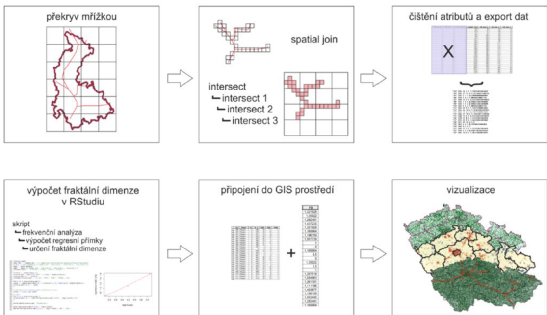
Obr. 3.6 Vlastný přístup doktora Pászta pri výpočte fraktálnej dimenzie cestnej siete (zdroj: Pászto, 2015)
