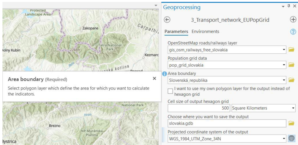
Obr. 4.3.3 Uživatelské rozhranie nástroja v ArcGIS Pro (autor: A. Tóth).
