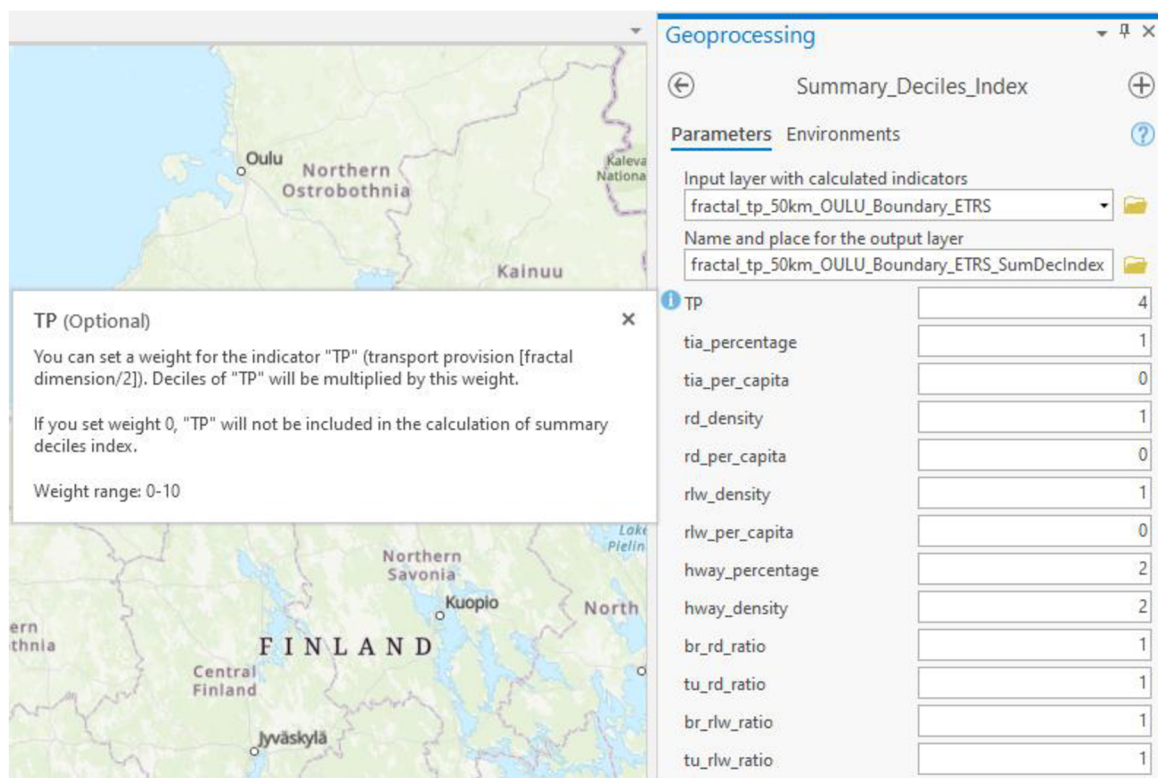
Obr. 4.6.1 Uživatelské rozhranie nástroja v ArcGIS Pro (autor: A. Tóth).
