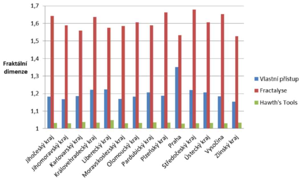
Obr. 3.7 Fraktálna dimenzia cestnej siete krajov ČR podľa použitých postupov výpočtu (zdroj: Pászto, 2015)
