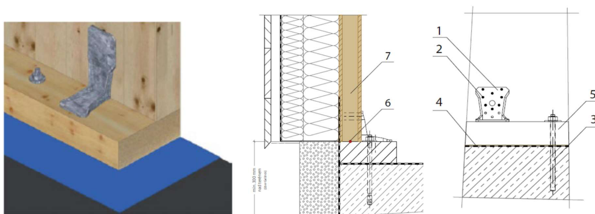
Obrázek 16 – Detail ND121, kotvení obvodové stěny ke zděné části domu (zdroj Novatop-System)
