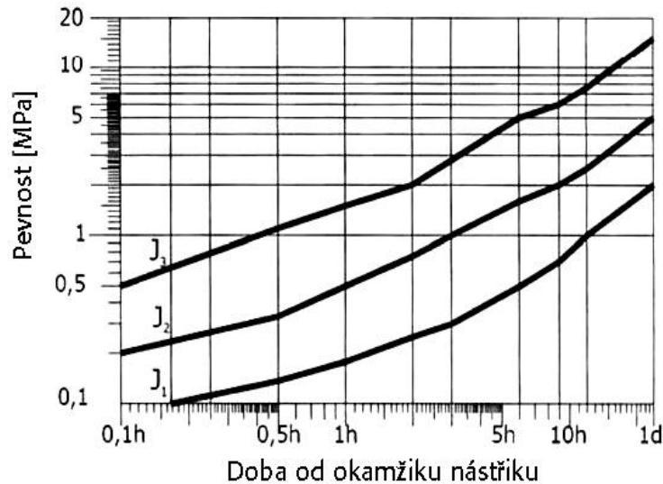
Obrázek 6: Obory nárůstu pevnosti mladého stříkaného betonu [1]
