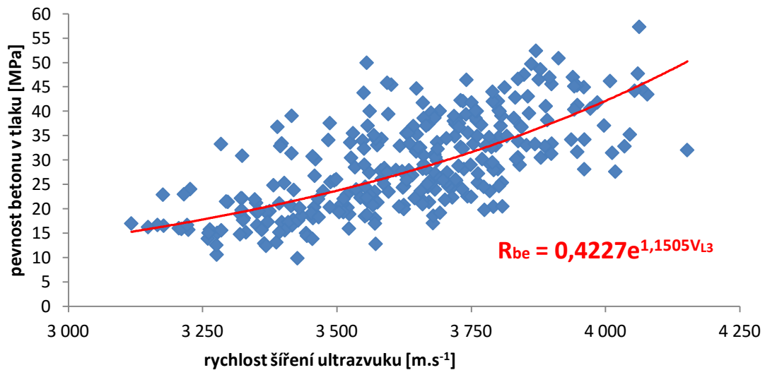
Graf 12: upravený vztah pro výpočet informativní pevnosti v tlaku na základě pevnosti v tlaku a rychlosti šíření ultrazvuku
