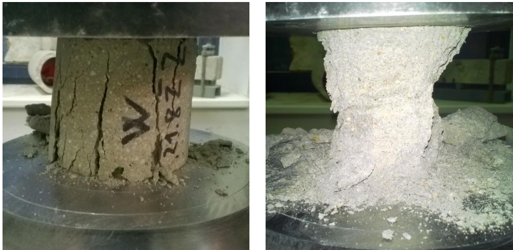
Obrázek 22: průběh zkoušky pevnosti v tlaku
