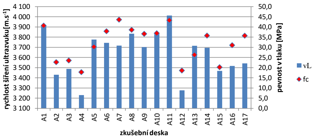
Graf 6: průměrná rychlost šíření ultrazvukového impulzu a pevnost v tlaku u jednotlivých zkušebních deskách
