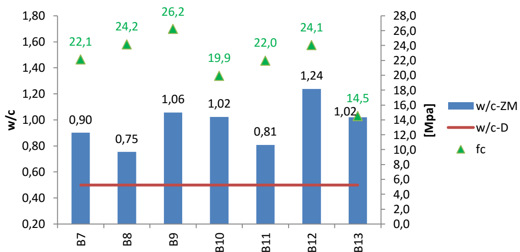
Graf 20: doporučený vodní součinitel, stanovený vodní součinitel, pevnost v tlaku
