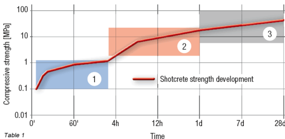
Obrázek 8: Grafické znázornění rozdělení metod pro měření pevnosti [Dr. Lindlar, B., CPE Jahn, M. Method Statement Strength Measurement of Shotcrete [online]. 2. verze, 2010-03-10 [cit. 2012-09-10] Dostupné z < http://www.sika.com/content/dam/Corporate/Microsite_Shotcrete/pdf/Method%20Statement%20Shotcrete%20Testing%20.pdf >]
