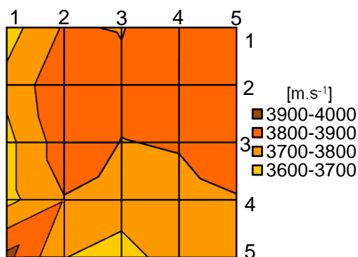
Graf 15 Rychlost průchodu ultrazvukového impulsu při polopřímém měření I.
