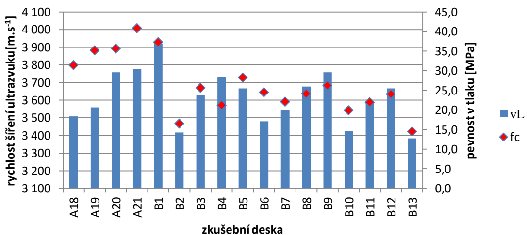
Graf 7: průměrná rychlost šíření ultrazvukového impulzu a pevnost v tlaku u jednotlivých zkušebních deskách
