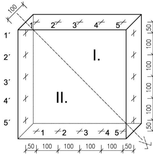
Obrázek 23: rozměření měřících bodů
