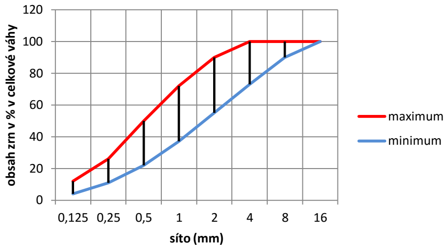
Obrázek 7: tělesa doporučené pásmo zrnitosti pro stříkaný beton [1]
