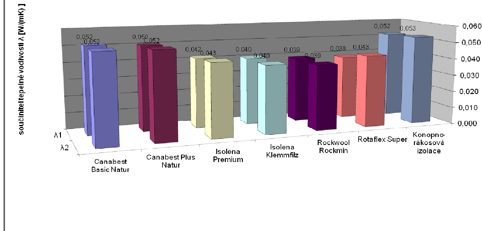
Graf 5 - Změna součinitele tepelné vodivosti \lambda před a po zkoušce krátkodobé nasákavosti \lambda_1 ..... průměrný součinitel tepelné vodivosti vzorku před ponořením \lambda_2 ..... průměrný součinitel tepelné vodivosti vzorku po ponoření a následném vysušení
