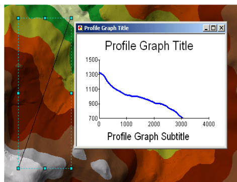
Obr. 14: Výškový profil [19]
