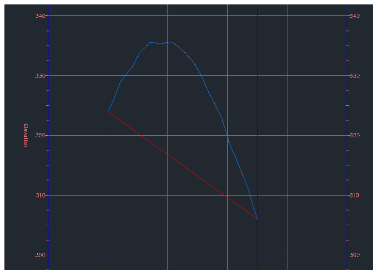
Obr. 48: Profil terénu
