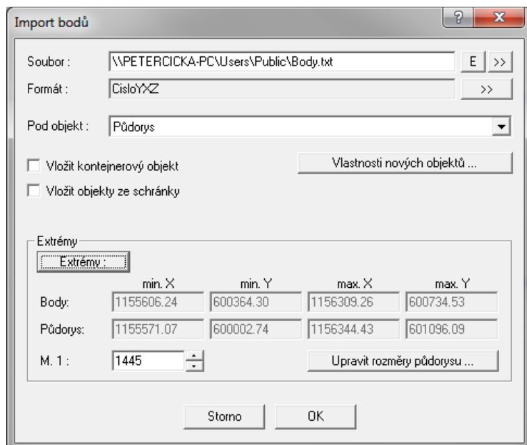
Obr. 63: Import bodov
