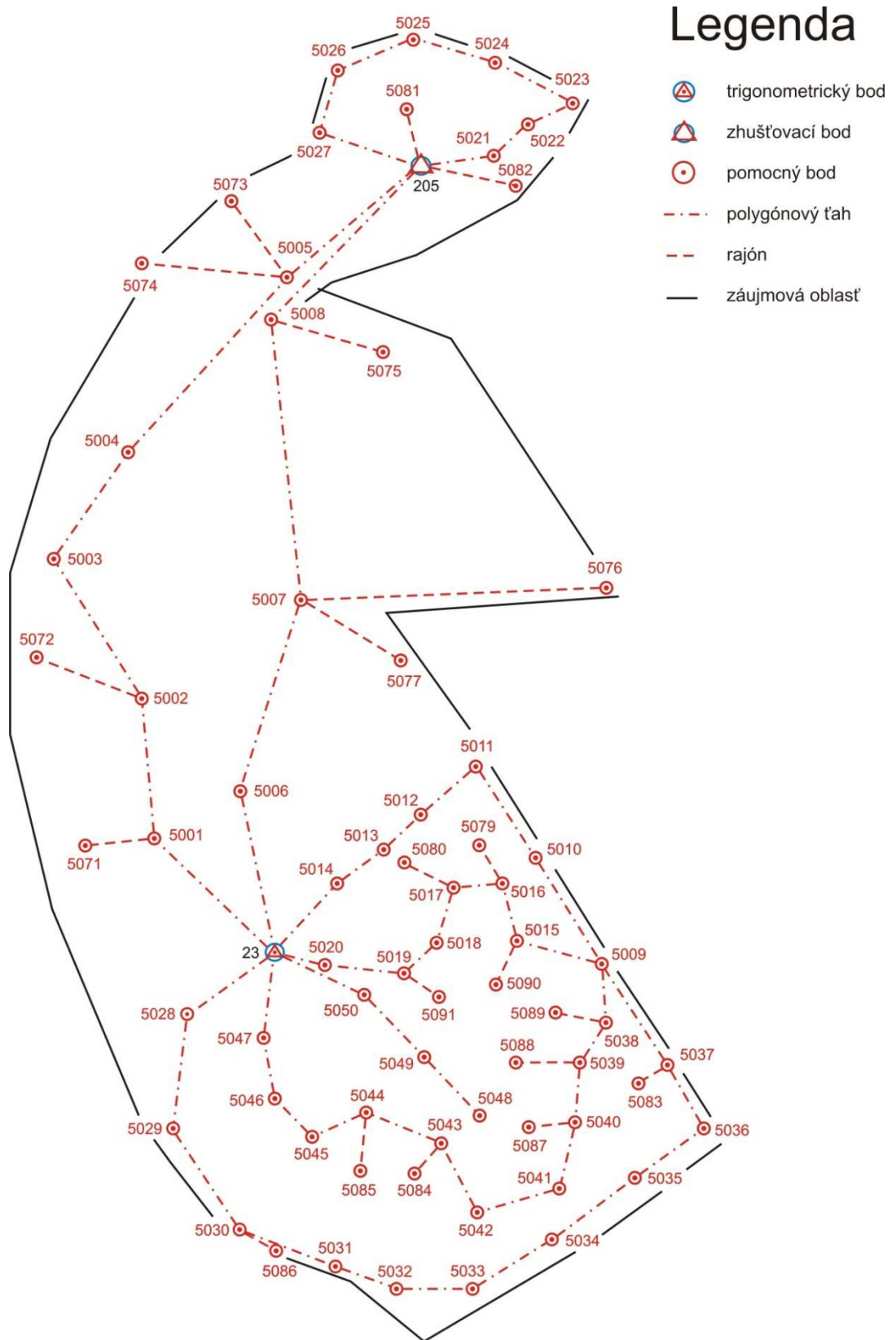
Obr. 24: Schéma meračskej siete a zúčtovnej oblasti [27]
