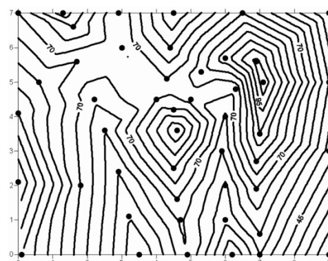
Metóda triangulácie
