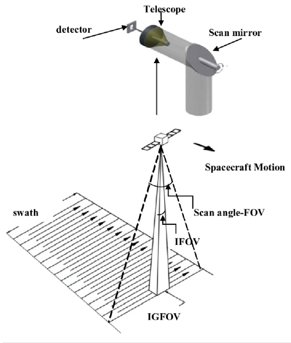
Obrázek 1: Whiskbroom senzor (Joseph, 2016)
