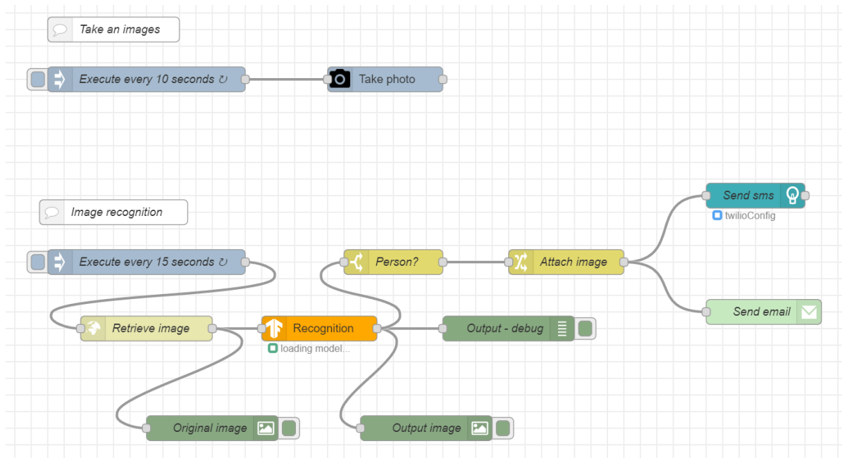
Obrázek 25 - Node-RED toky pro kamerový systém (vlastní zpracování)
