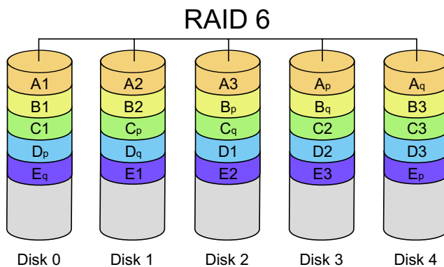
Obrázek 3.10 RAID 6 [18]
