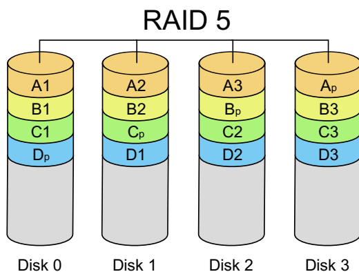
Obrázek 3.9 RAID 5 [18]
