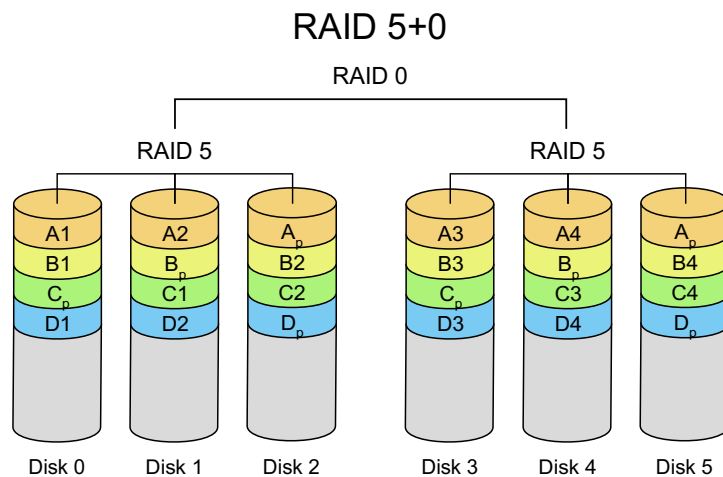
Obrázek 3.11 RAID 50 [18]
