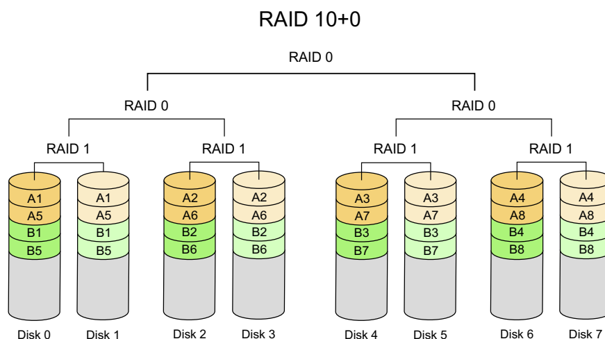
Obrázek 3.13 RAID 100 [18]
