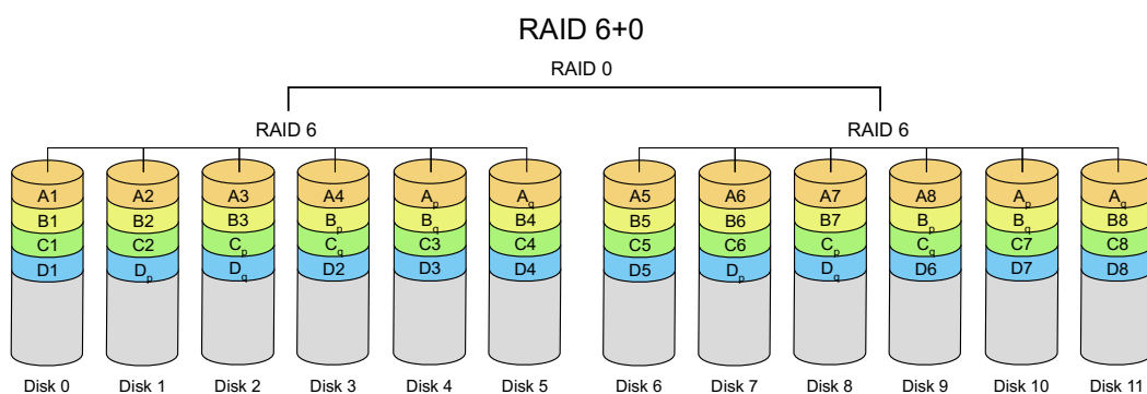
Obrázek 3.12 RAID 60 [18]
