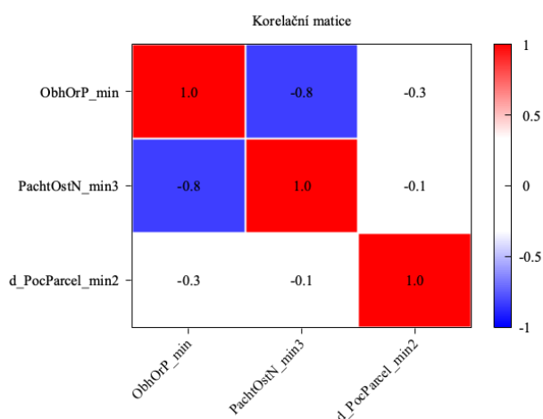
Obrázek 5: Korelační matice
