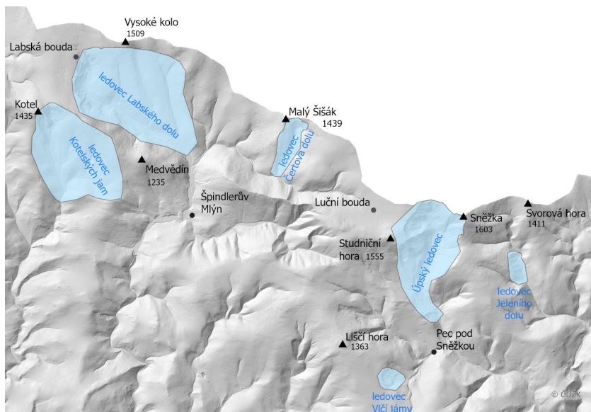
Obrázek 12: Předpokládaný rozsah würmského zalednění Krkonoš (ENGEL 2007, ČÚŽK 2023b, ČÚŽK 2024a, ČÚŽK 2024b, vlastní zpracování)
