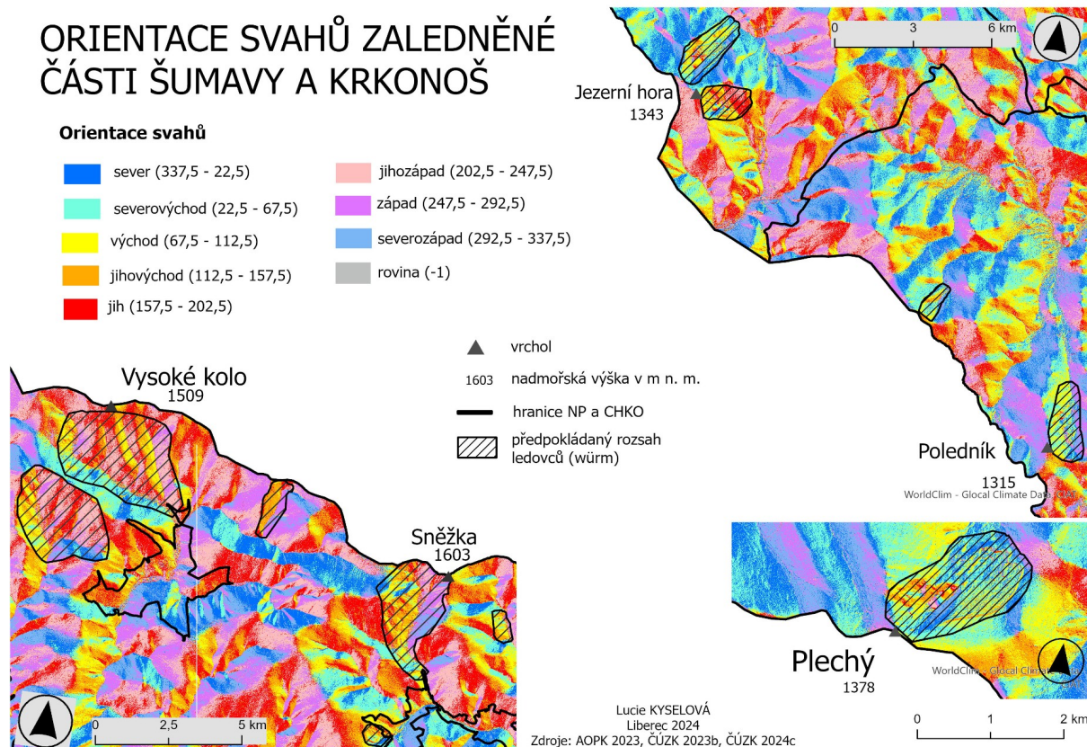
Obrázek 18: Orientace svahů v zámjových územích (AOPK 2023, ČÚZK 2023b, ČÚZK 2024c, vlastní zpracování)
