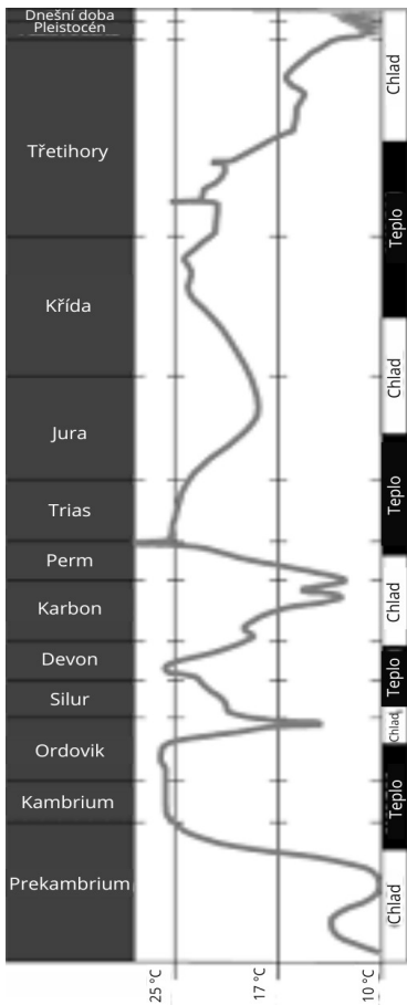
Obrázek 1: Vývoj klimatu v historii Země (Scotese 2015, upraveno)
