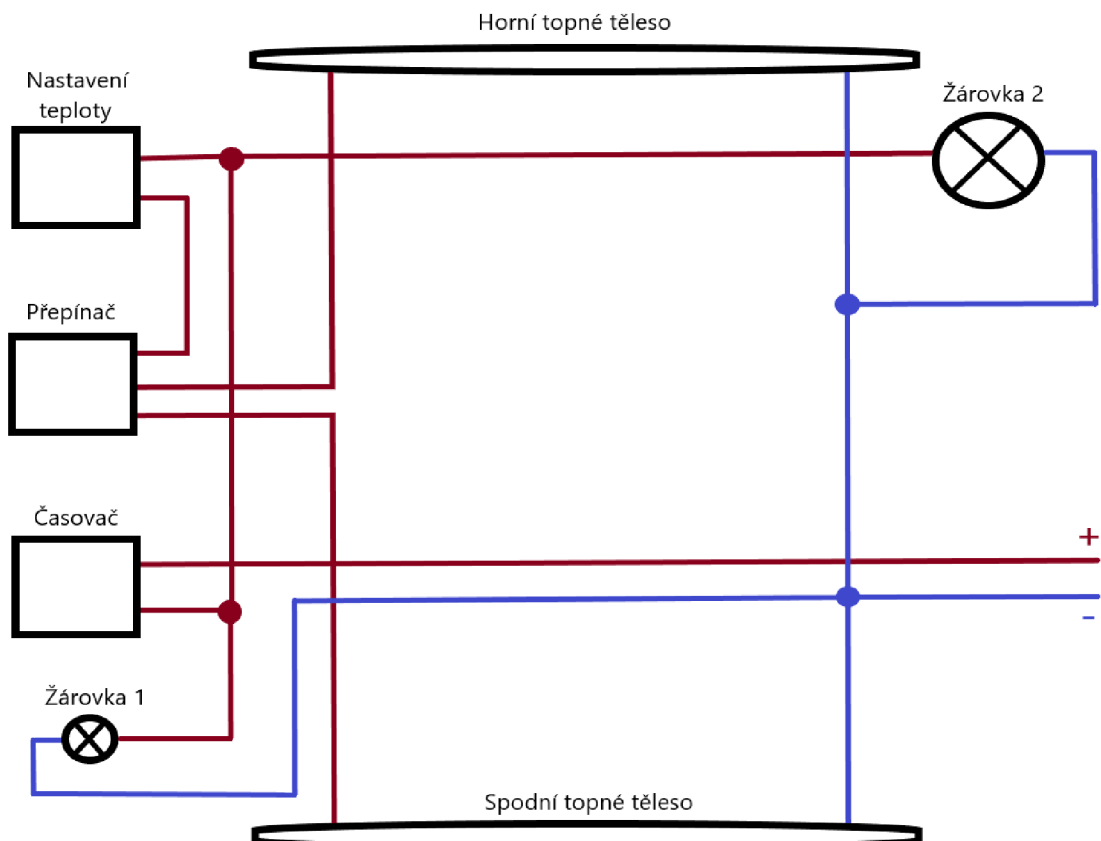
Obrázek 19: Schéma původního zapojení
