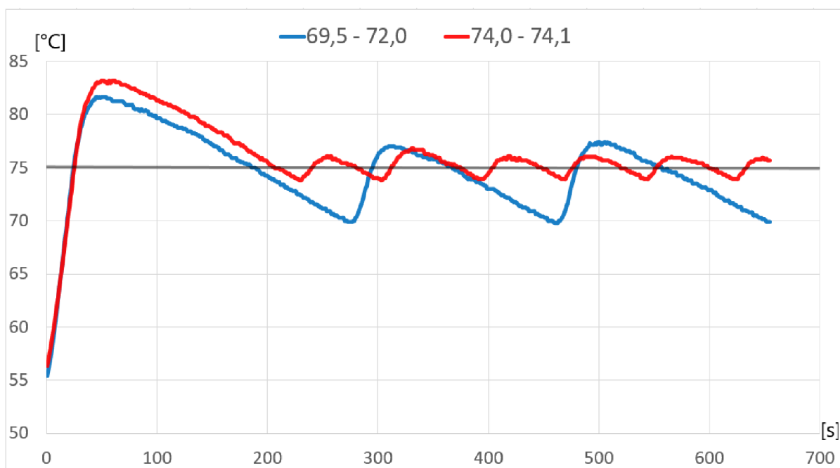
Obrázek 27: Průběh dvoustavové regulace (obě topná tělesa)
