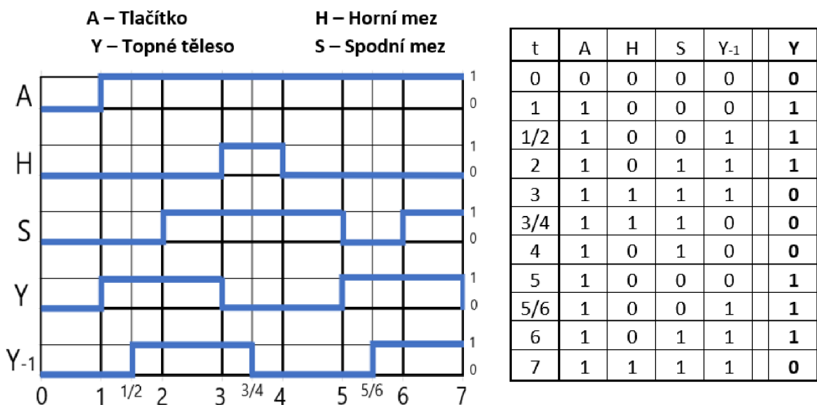
Obrázek 23: Postup řešení dvoustavové regulace
