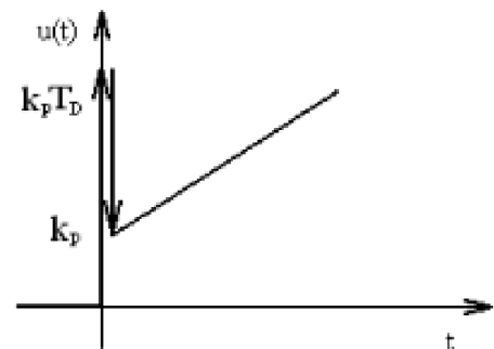
Obrázek 5: Přechodová charakteristika PID regulace [7]
