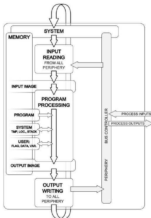
Obrázek 8: Princip PLC [12]
