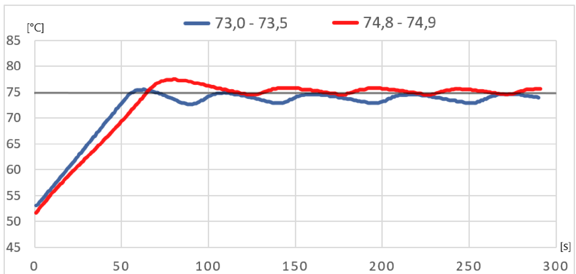
Obrázek 26: Průběh dvoustavové regulace (horní topné těleso)
