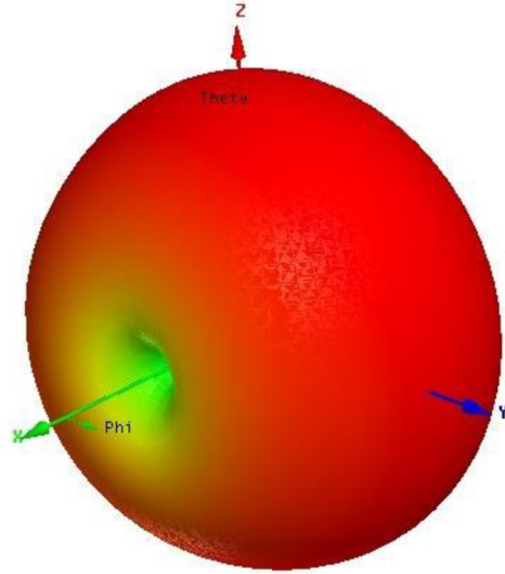
Obrázek 5.6 3D směrová charakteristika antény; anténa ve volném prostoru.
