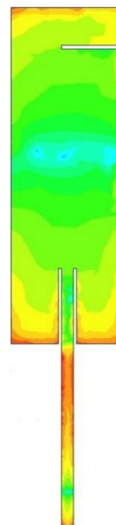
Obrázek 5.4 Rozložení proudů na anténě; anténa ve volném prostoru.
