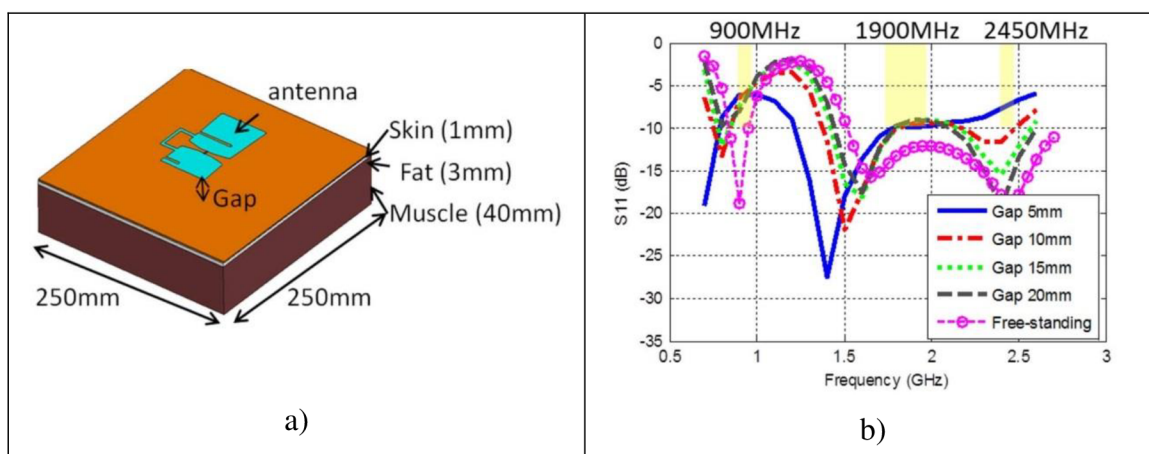
Obrázek 1.2 Vyšivaný nesymetrický dipól na modelu lidské tkáně (vlevo). Kmitočtový průběh velikosti činitele odrazu na vstupu antény v závislosti na vzdálenosti antény od fantomu (vpravo). Převzato z [1].
