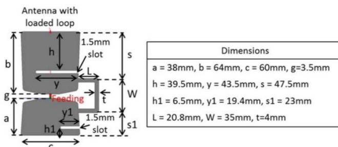
Obrázek 1.1 Vyšivaný nesymetrický dipól a jeho parametry. Převzato z [1].
