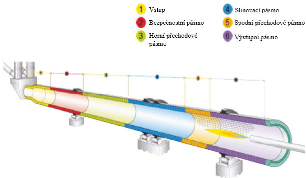
Obrázek 2.3: Rozdělení zón v cementářské rotační peci
