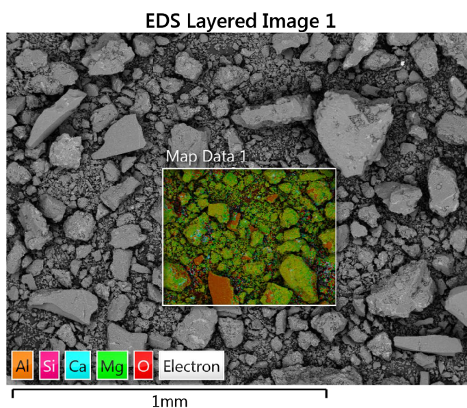
Obrázek 4.1: Oblast prvkové analýzy vzorku C1
