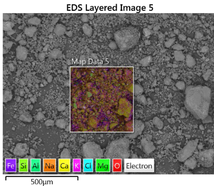
Obrázek 4.3: Oblast prvkové analýzy vzorku B2 při zvětšení 200×
