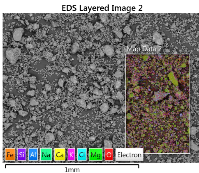
Obrázek 4.2: Oblast analýzy pro prvkovou mapu vzorku A4
