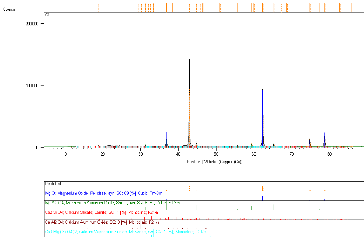
Obrázek 8.11: Fázové složení vzorku C1
