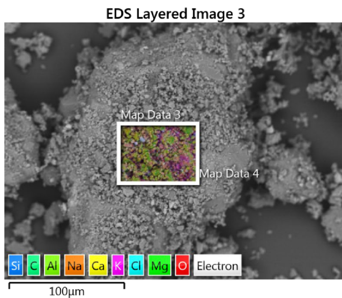
Obrázek 4.4: Oblast prvkové analýzy vzorku B2 při zvětšení 1000×
