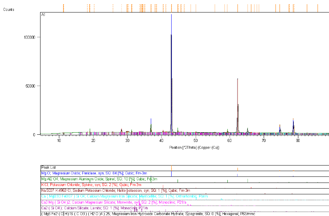
Obrázek 8.1: Fázové složení vzorku A1
