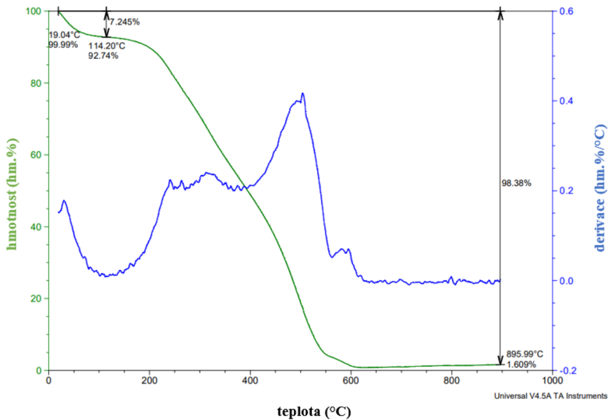
Obrázek 11: TGA HK 10 cm
