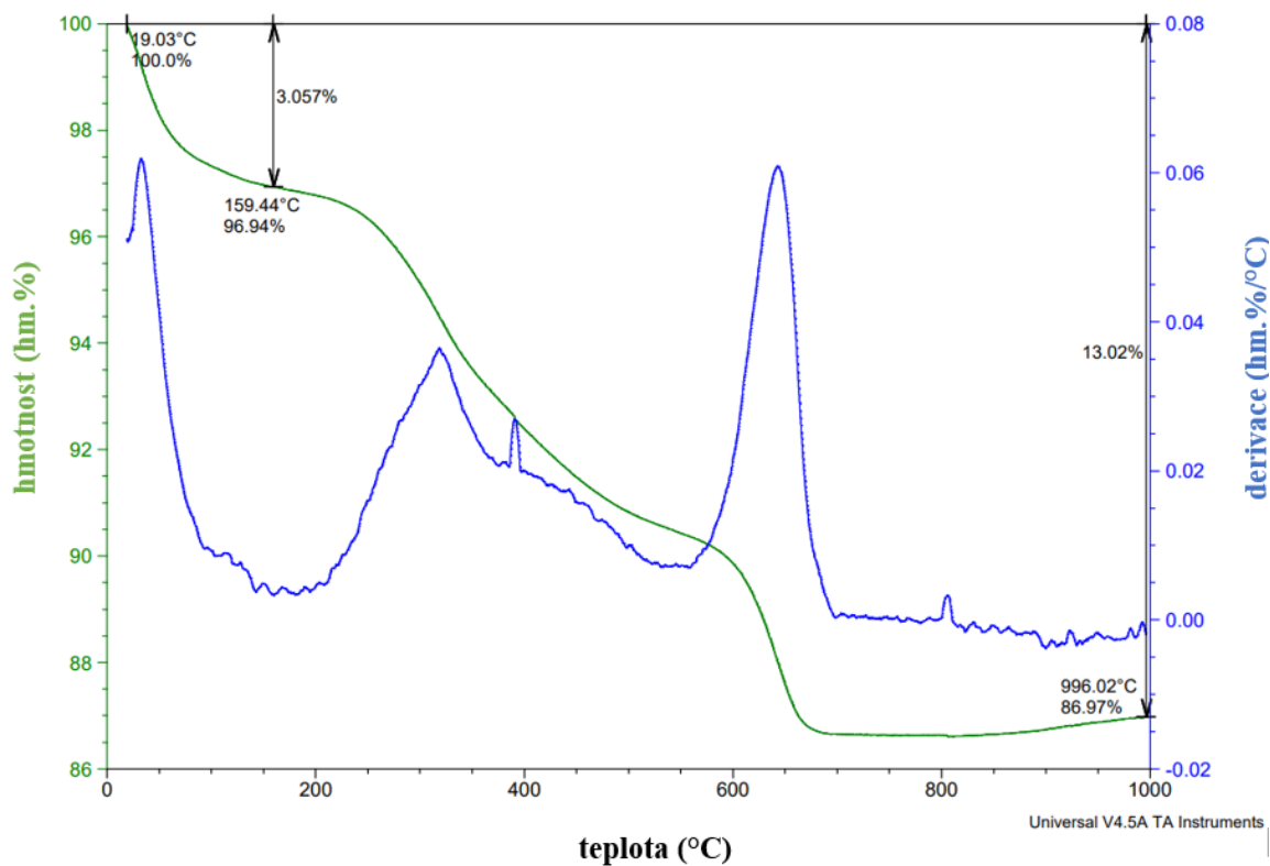
Obrázek 9: TGA pŕdy 10 cm
