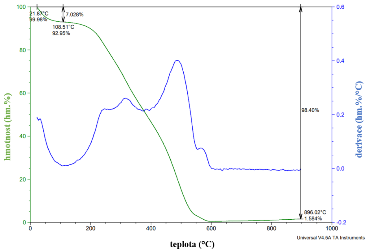
Obrázek 12: TGA HK 30 cm
