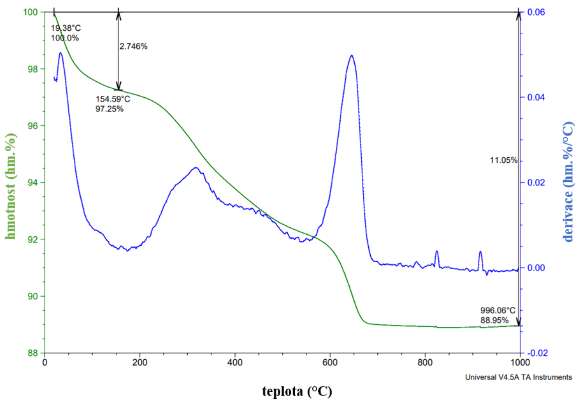
Obrázek 10: TGA pŕdy 30 cm
