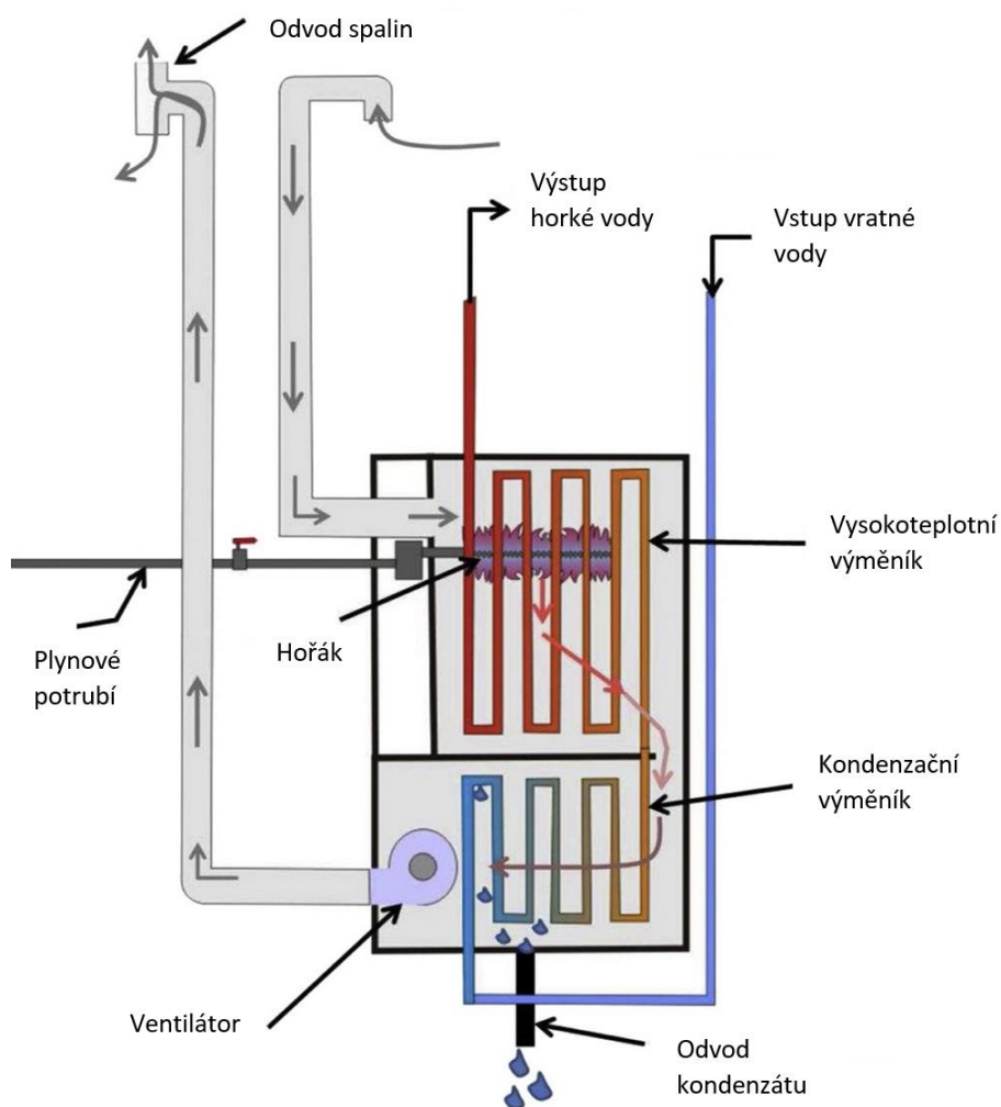
Obr. 5 Způsob konstrukce kondenzačního kotle [10]
