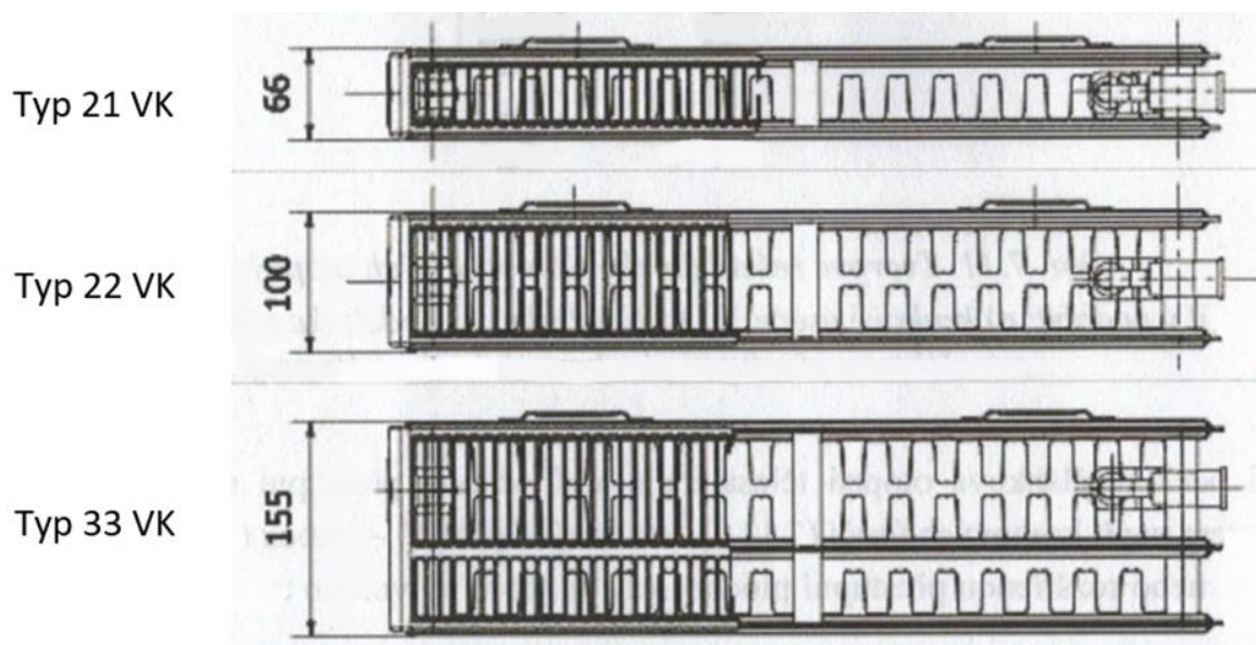
Obr. 2 Přehled základních typů deskových otopných těles [3]
