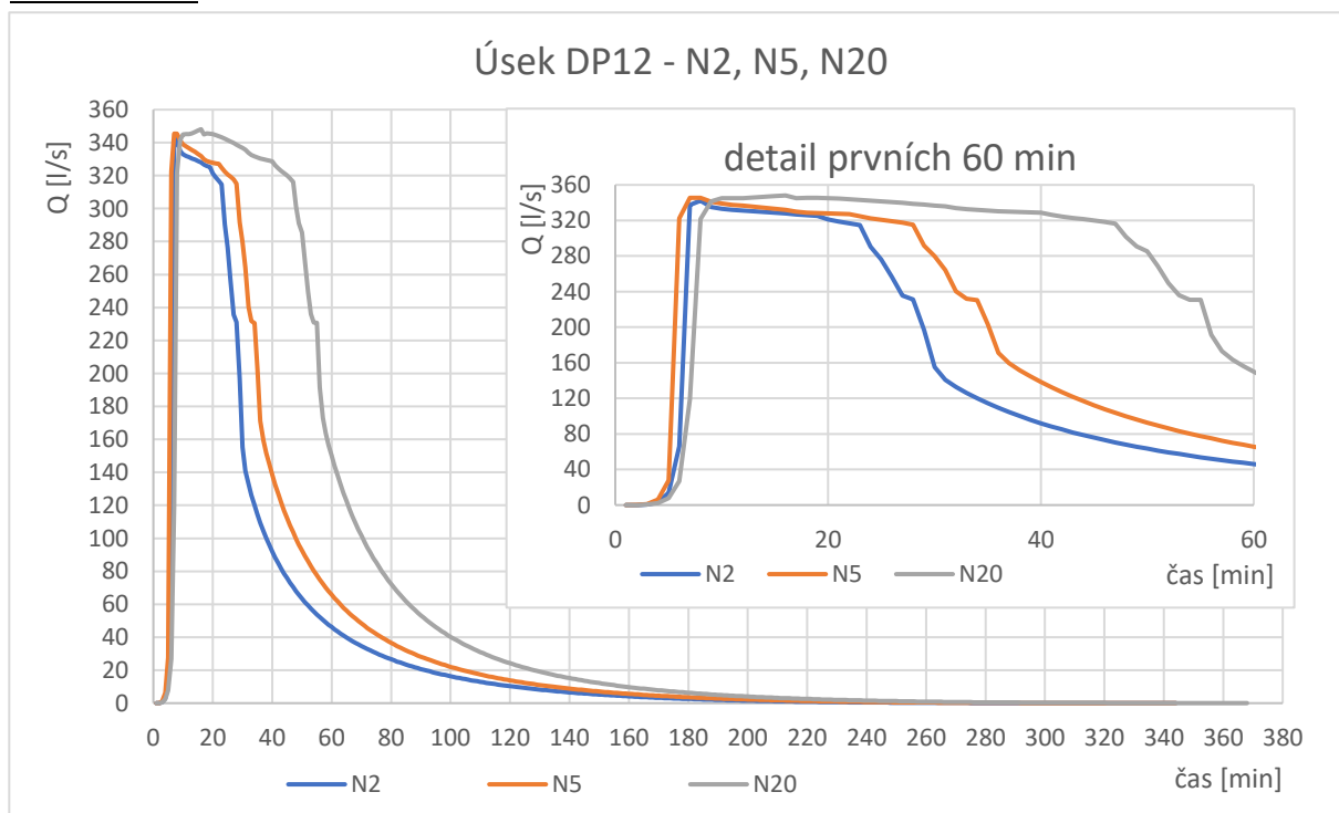
Obr. 4.26. Průtokové křivky úseku DP12 – plánovaný rozvoj
