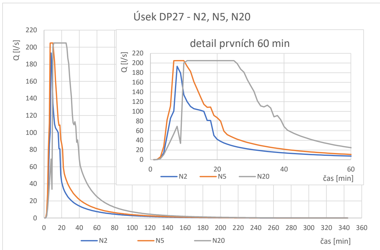
Obr. 4.12. Průtokové křivky úseku DP27 – stávající stav
