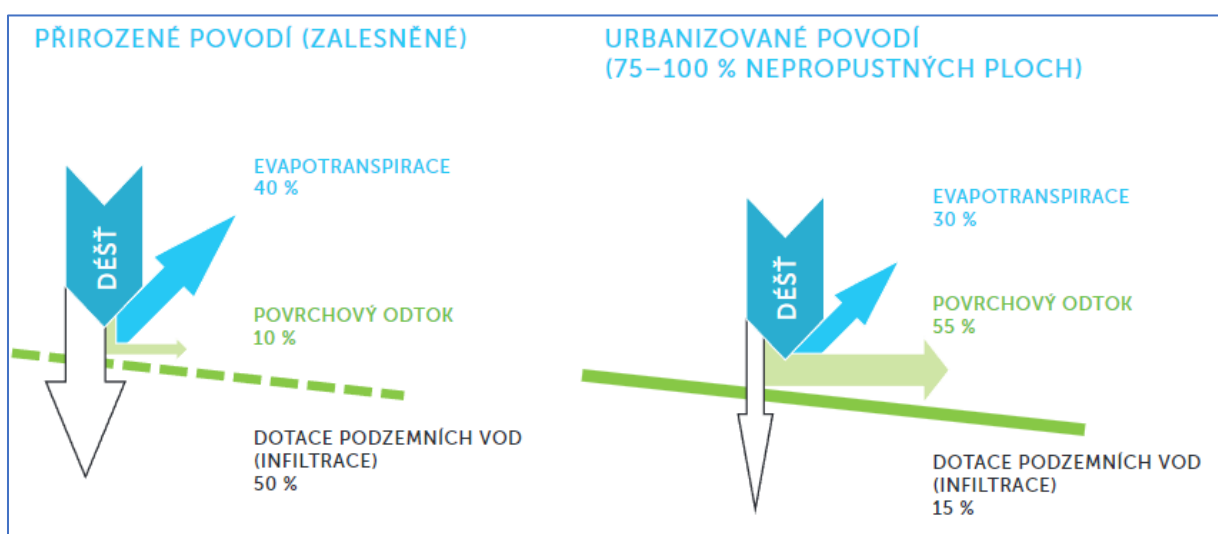
Obr. 3.6. Porovnání chování dešťové srážky v přirozeném a urbanizovaném povodí [17]
