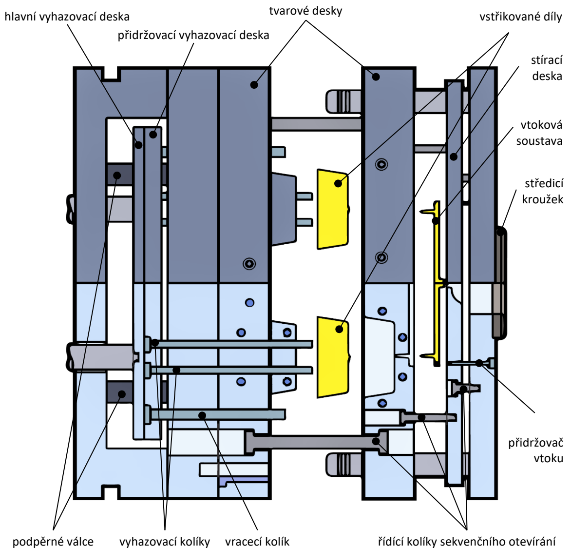
Obr. 2.7 Schéma otevřené třideskové vstřikovací formy
