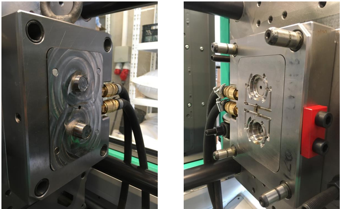
Obr. 4.37 Upnutá vstřikovací forma na vstřikovacím stroji
