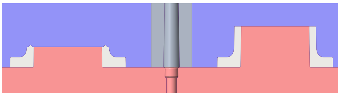
Obr. 3.4 Zaformování dílů, dělení formy
