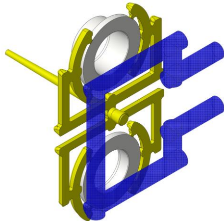
chladicí okruh pohyblivé poloviny
