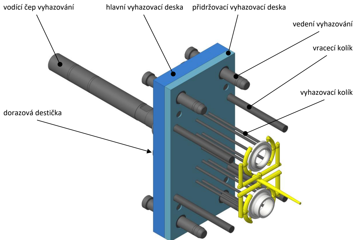
Obr. 4.30 Navržený systém vyhazování
