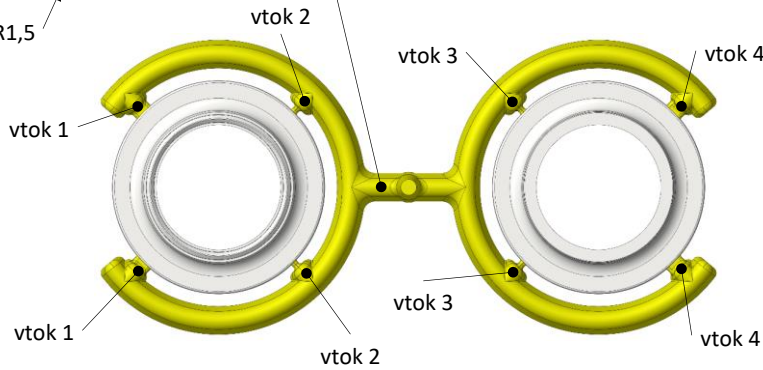
Obr. 4.14 Rozměry vtokového systému – varianty c)
