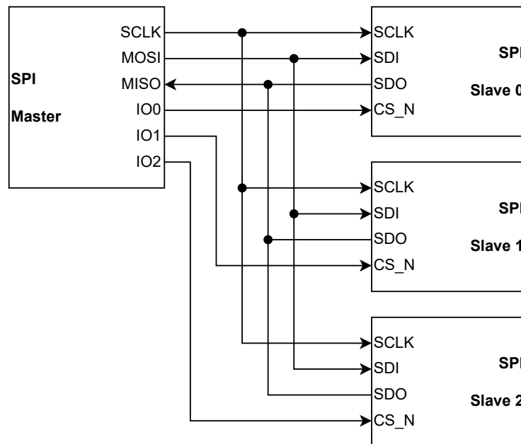
Obr. 4.1: SPI zapojení Master a Slave zařízení
