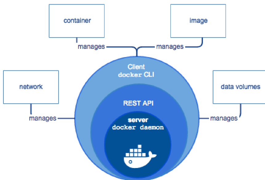
Obrázek 10 - Docker engine. Zdroj: (95)
