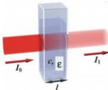
Obr. 20 Průchod záření kyvetou [136]
