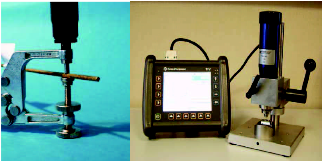
Obr. 3.4 Příslušenství k mobilním tvrdoměrům, zleva kleště pro měření malých dílu a stojánek s prizma pro měření válcových ploch (6)
