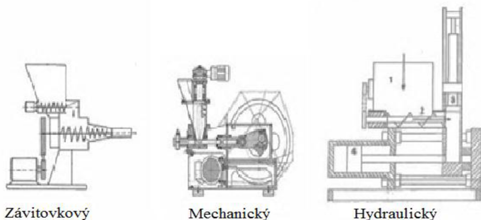
Obr. 5.6 Základné konštrukcie briketovacích lisov [11]
