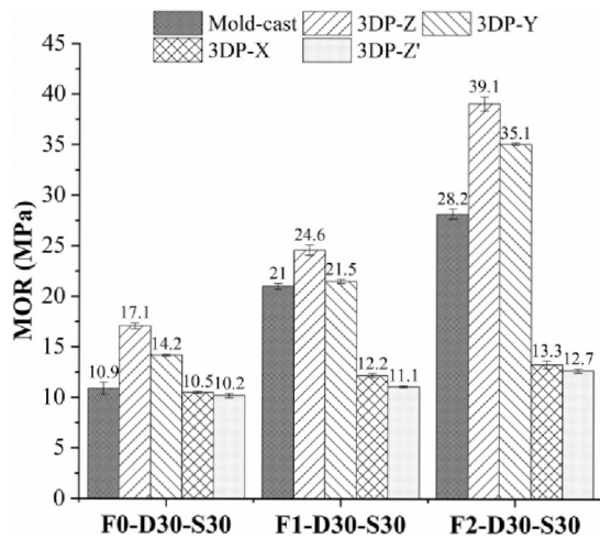
(c) Modulus lomu (MOR) v závislosti na dávce vláken.
