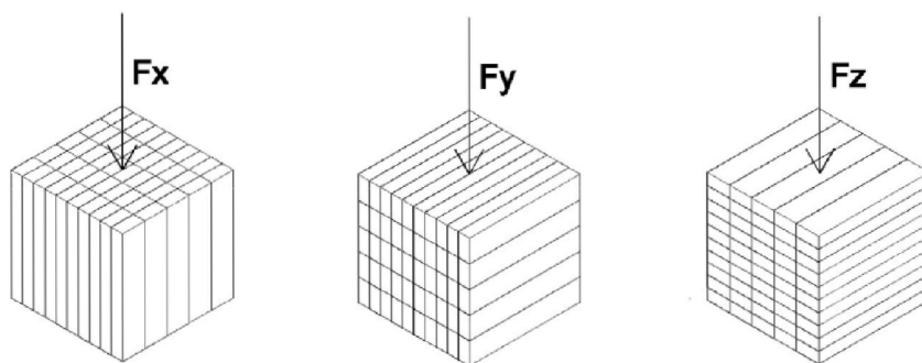
(d) Vyřezaný vzorek z 3D tisku a směry zatěžování pro pevnost v tlaku. [11]
