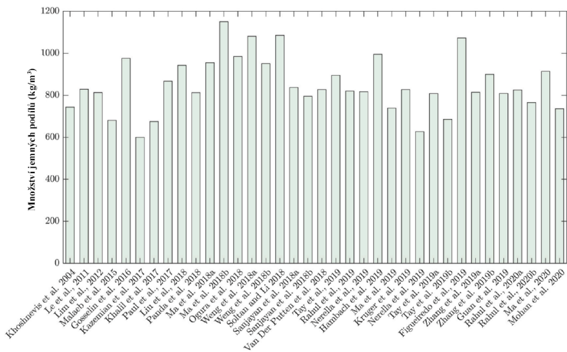
Obrázek 5.18: Množství pojiva v různých 3D recepturách. V grafu je vyneseno celkové množství pojiv v recepturách pro 3D tisk. [6]
