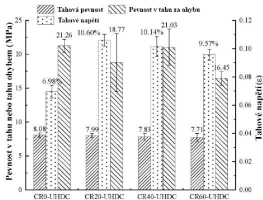
(b) Pevnost tahová a v tahu za ohybu a tahové napětí.
