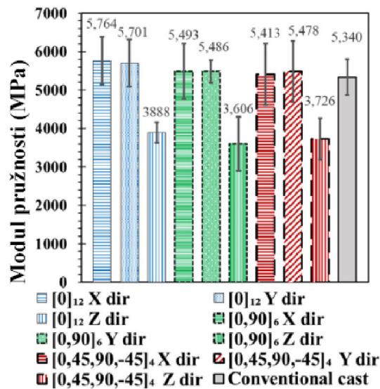
(c) Modul pružnosti různých směrů tisků a plnění.
