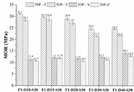
(b) Modulus lomu (MOR) v závislosti na velikosti trysky.
