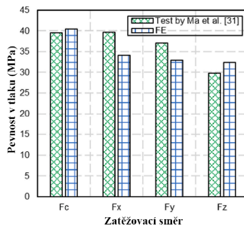
(b) Pevnost v tlaku simulace a reality - porovnání 2
