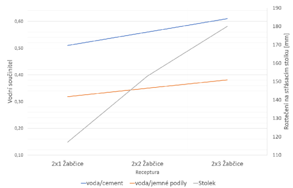
(c) Porovnání receptury s kamenivem Žabčice 0-4.
