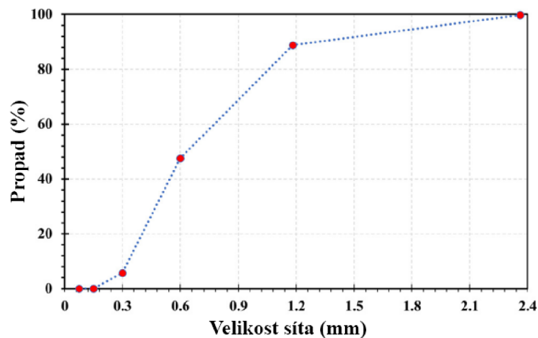
Obrázek 5.4: Křivka zrnitosti písku v receptuře 3. [9]
