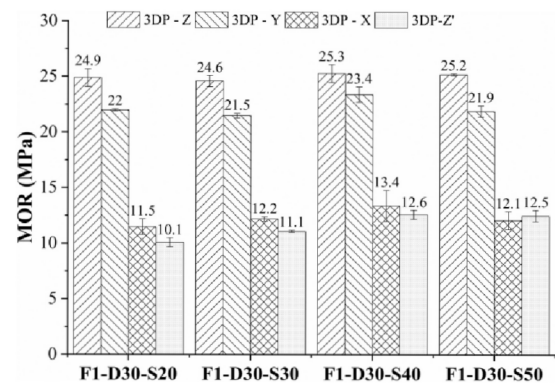
(d) Modulus lomu (MOR) v závislosti na rychlosti tisku.
