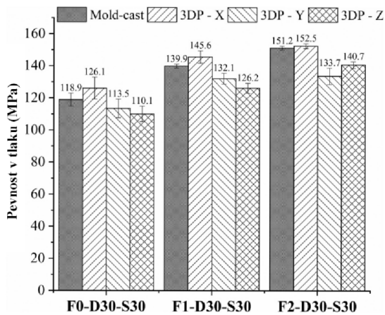
(a) Pevnost v tlaku v závislosti na dávce vláken.
