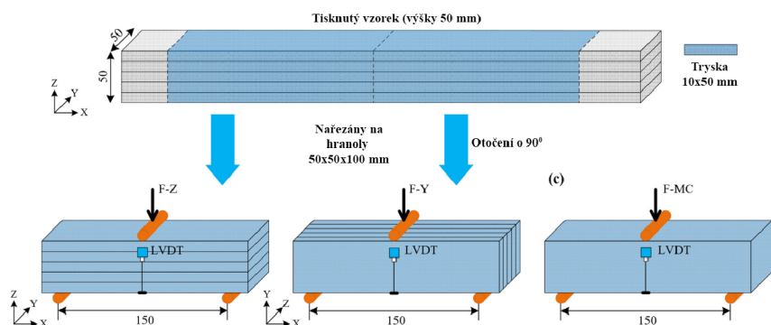
(e) Vyřezaný vzorek z 3D tisku a směry zatěžování pro pevnost v ohybu. [10]
