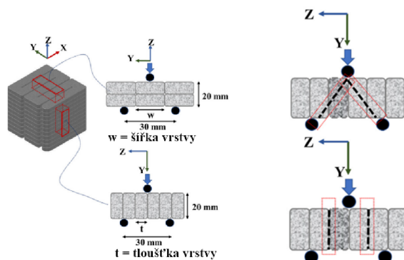
(c) Vyřezaný vzorek z 3D tisku a směry zatěžování pro pevnost v ohybu. [9]
