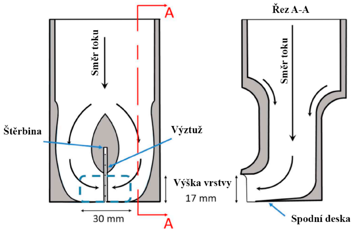
Obrázek 6.15: Řez tryskou. [16]
