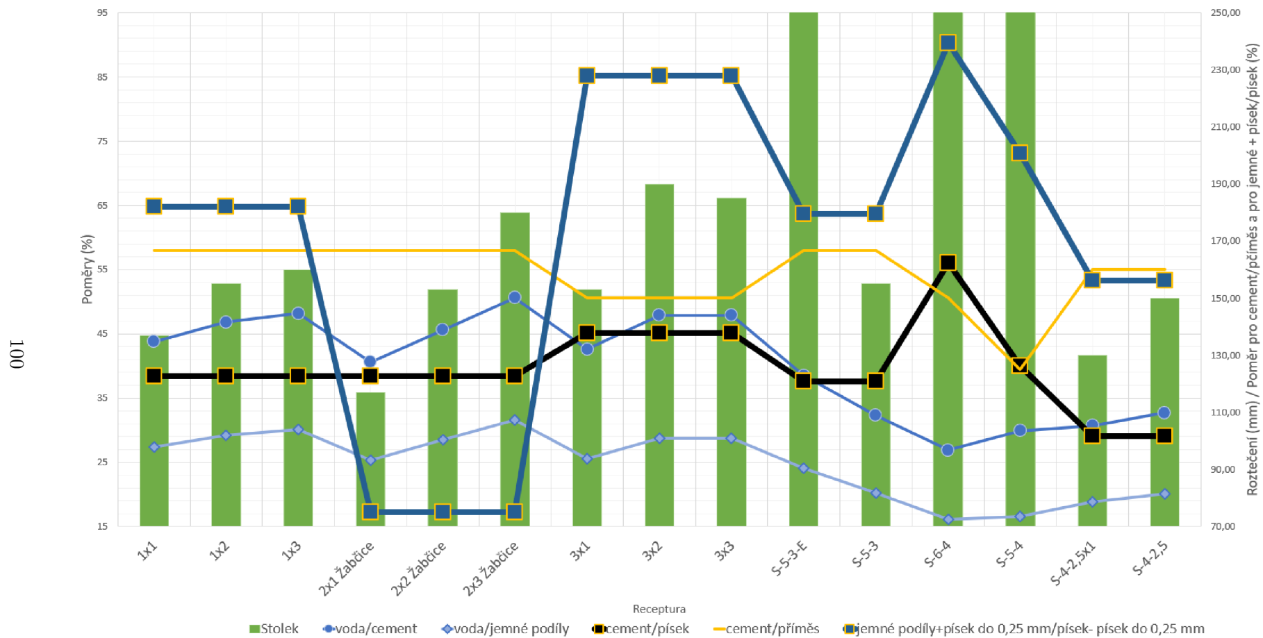
Obrázek 7.3: Porovnání vodních součinitelů a poměrů jemných podílů vůči písku s roztečením.
