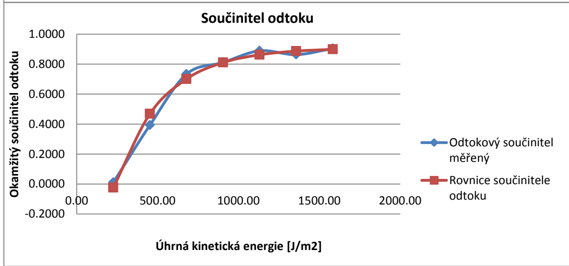
Obr. 24. Ombrologická křivka a součinitel odtoku pro i = 1,52 \text{ m/min} , W_{k1} 40
