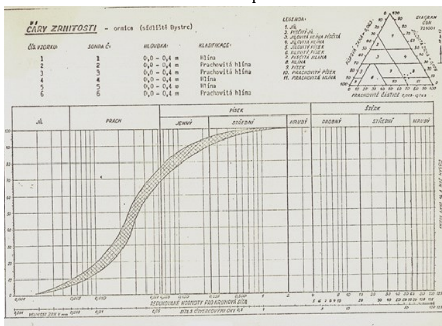
Obr. 2. Křivka zrnitosti - původní vzorek (ornice) 14
