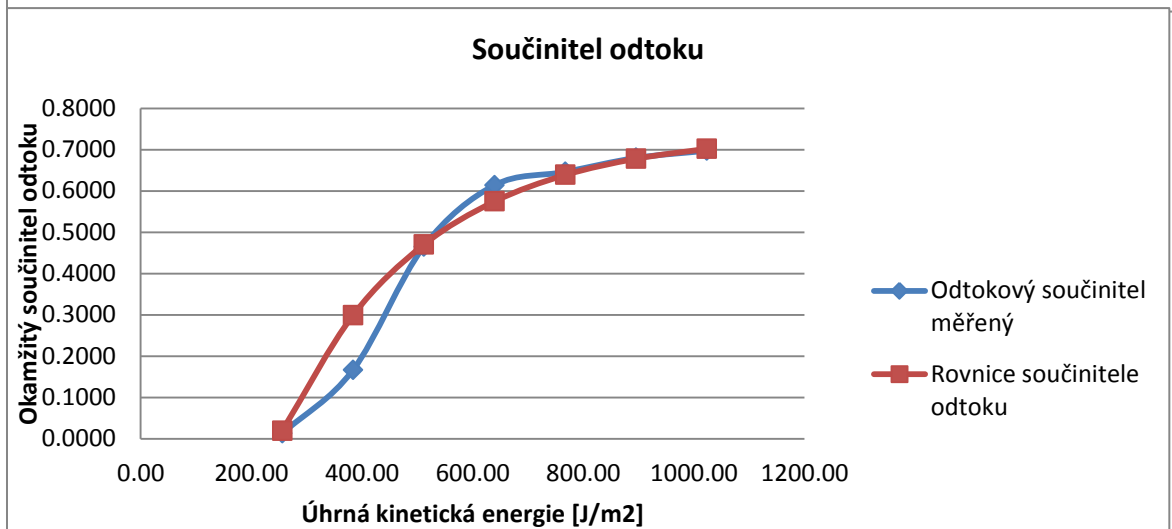
Obr. 30. Ombrologická křivka a součinitel odtoku pro i = 0,96 \text{ mm/min} , w_{k2} 46
