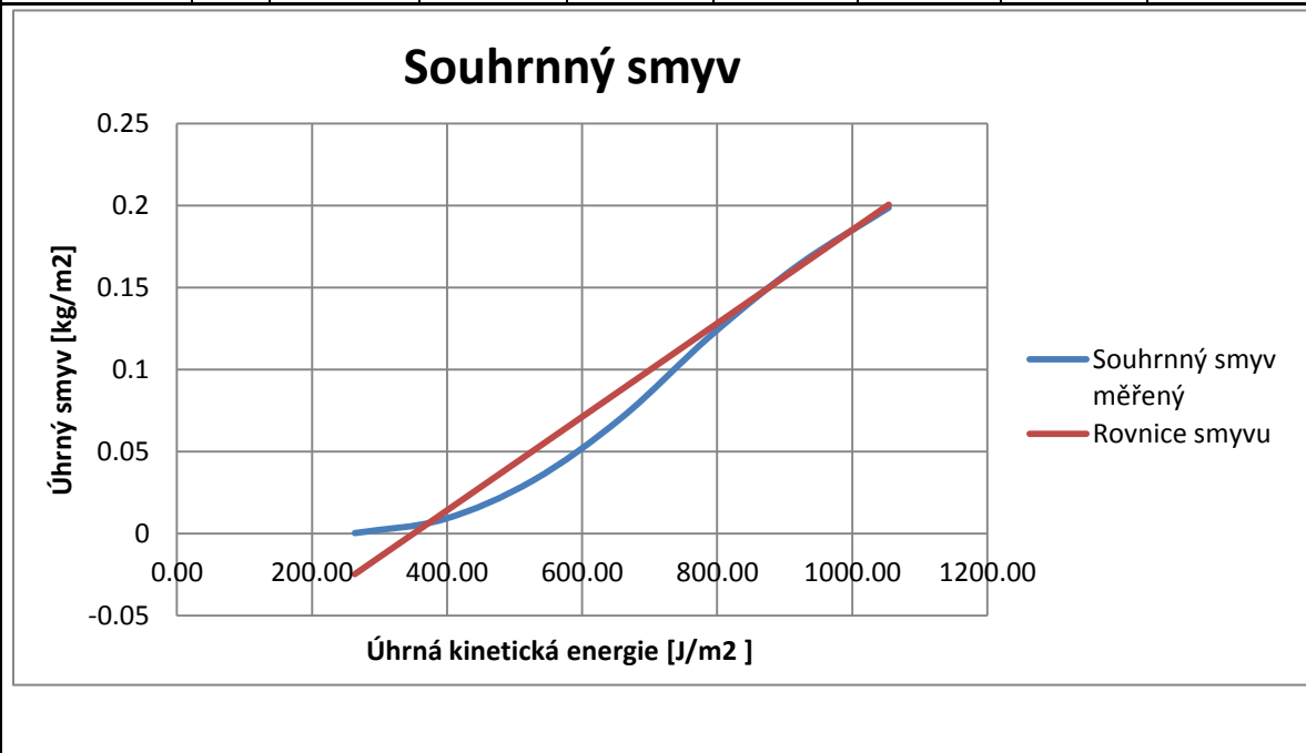
Obr. 25. Souhrnný smyv pro i = 0,96 \text{ mm/min} , w_{kl} 41
