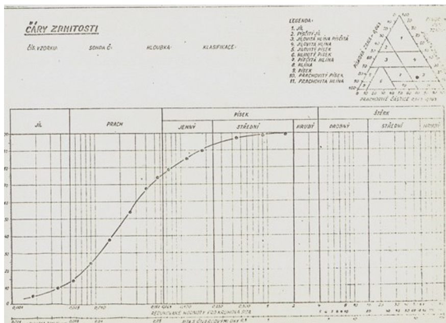
Obr. 1. Křivka zrnitosti – původní vzorek 13
