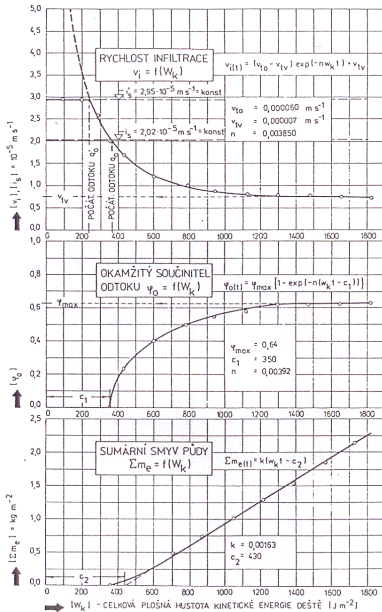
Obr. 35. Erozní vlastnosti půdy, i = 1.507 \text{ mm/min} 53
