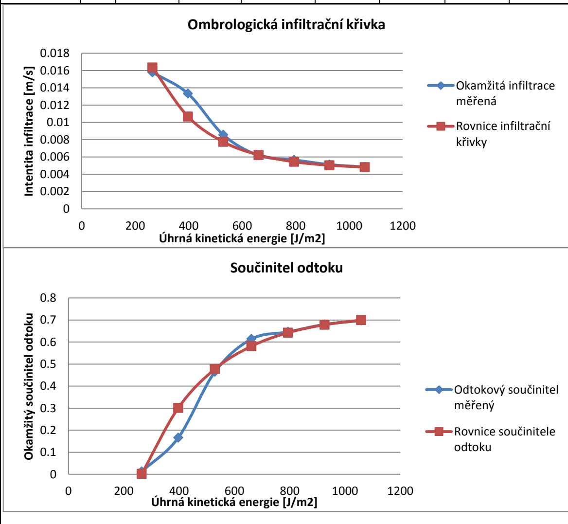
Obr. 26. Ombrologická křivka a součinitel odtoku pro i = 0,96 mm/min, w_{kl} 42
