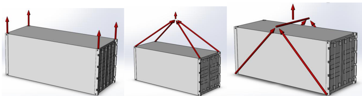
Obr. 4.5 Způsoby zdvihání a) zdvihání za horní část závěsným rámem, b) zdvihání za horní část lanovým závěsem, c) zdvihání za dolní část lanovým závěsem [vlastní obrázek]
