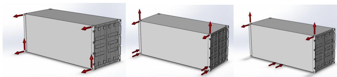
Obr. 4.6 Boční způsoby zdvihání a) způsob 1, b) způsob 2, c) způsob 3 [vlastní obrázek]
