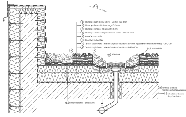
Obr. 161: řez zelené střechy (www.knaufinsulation.cz)
