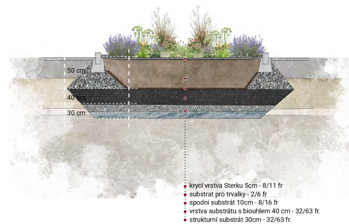
Obr. 160: řez trvalkového záhonu (autorská práce)
