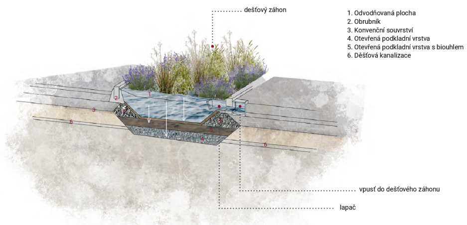
Obr. 159: řez dešťového záhonu (autorská práce)
