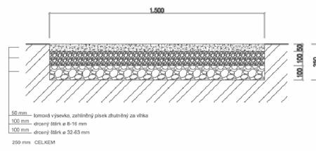
Obr. 163: řez mlatovou cestou Obr. 164: řez mlatovou cestou (autorská práce) (autorská práce)
