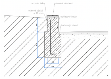
Obr. 162: řez betonovou lavicí (autorská práce)
