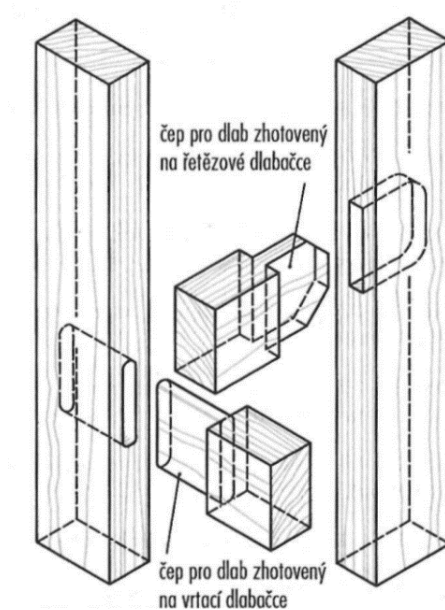
Obrázek 19 - Spoj na čep a dlab (Nutsch, 2012)
