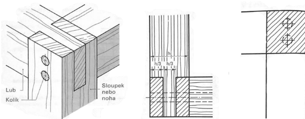
Obrázek 17 - Spoj na čep a rozpor (Nutsch a kol., 2007)
