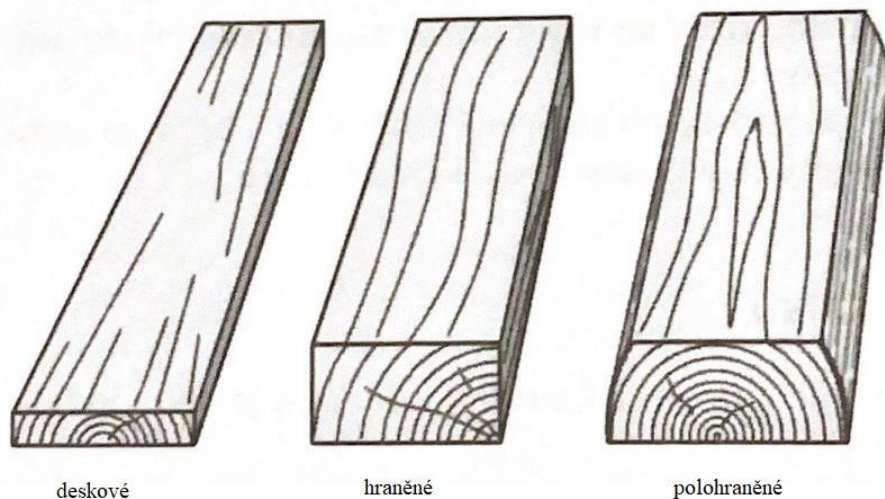
Obrázek 7 - Dělení řeziva dle příčného průřezu (Muzikář, 2008)
