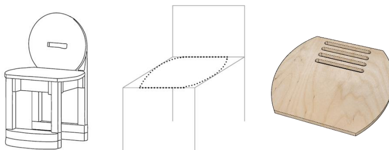
Obrázek 27 - Varianta sedáku odpovídající tvaru židle od firmy Little Design s.r.o.
