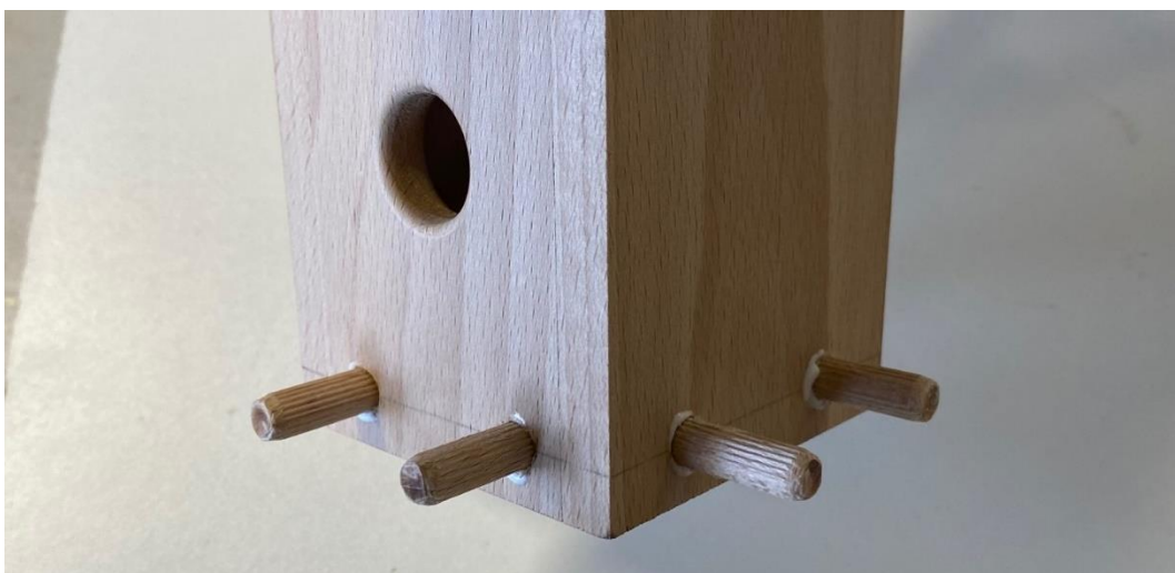
Obrázek 82 - Spojení dna s dutou nohou pomocí vlepěných kolíků o rozměru 8 x 40 mm
