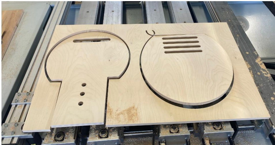
Obrázek 61 - Výroba sedáku a opěradla na CNC
