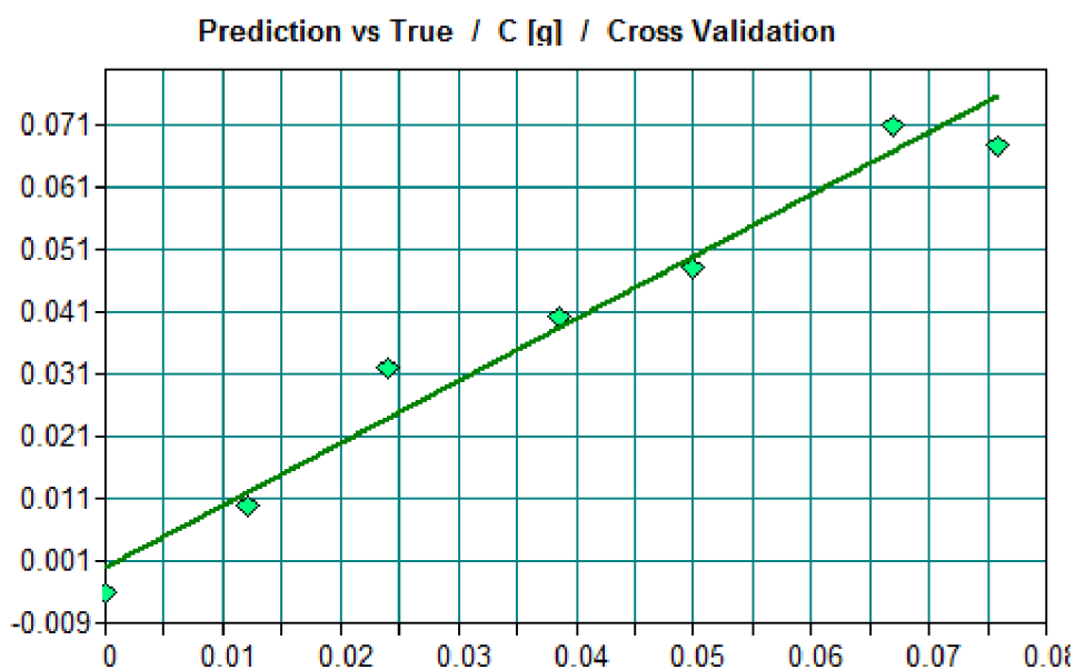
Obrázok 30: Validačný model pre sériu M34+PET s využitím hmotnosti uhlíku
