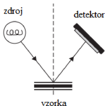
Obrázok 11: FTIR usporiadanie
