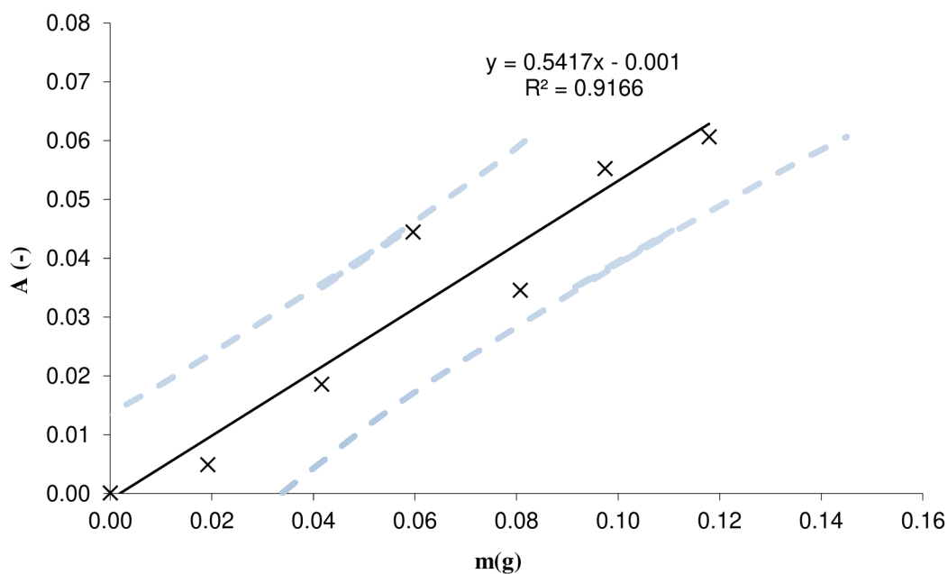
Graf 1: Kalibračná priamka závislosti absorpcie od hmotnosti plastu pre sériu M31+PET a prvý pík
