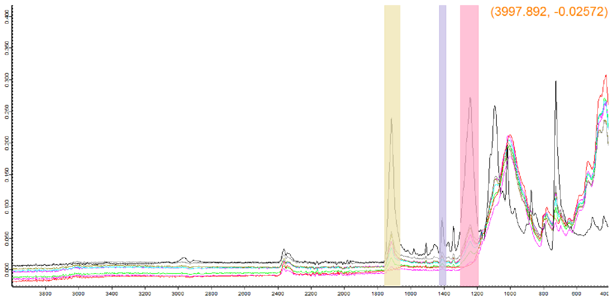
Obrázok 16: ATR absorpčné spektrá série M31+PET, čistej M31 (červená) a čistého PET (čierna)
