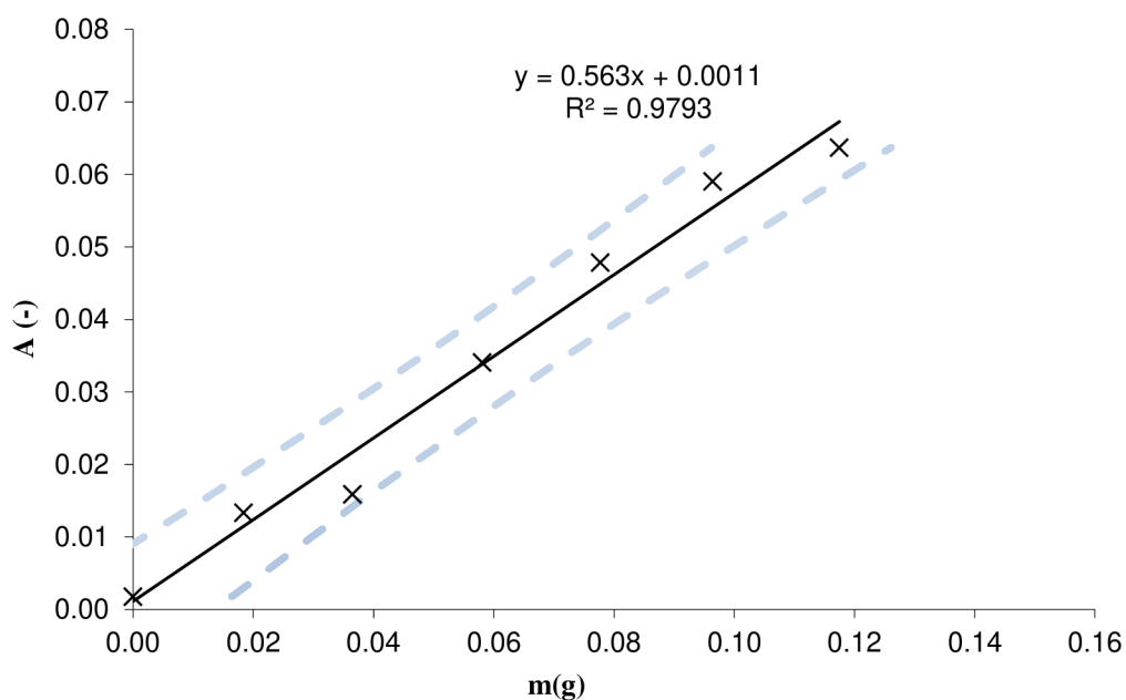
Graf 2: Kalibračná priamka závislosti absorbancie od hmotnosti plastu pre sériu M33+PET a prvý pík
