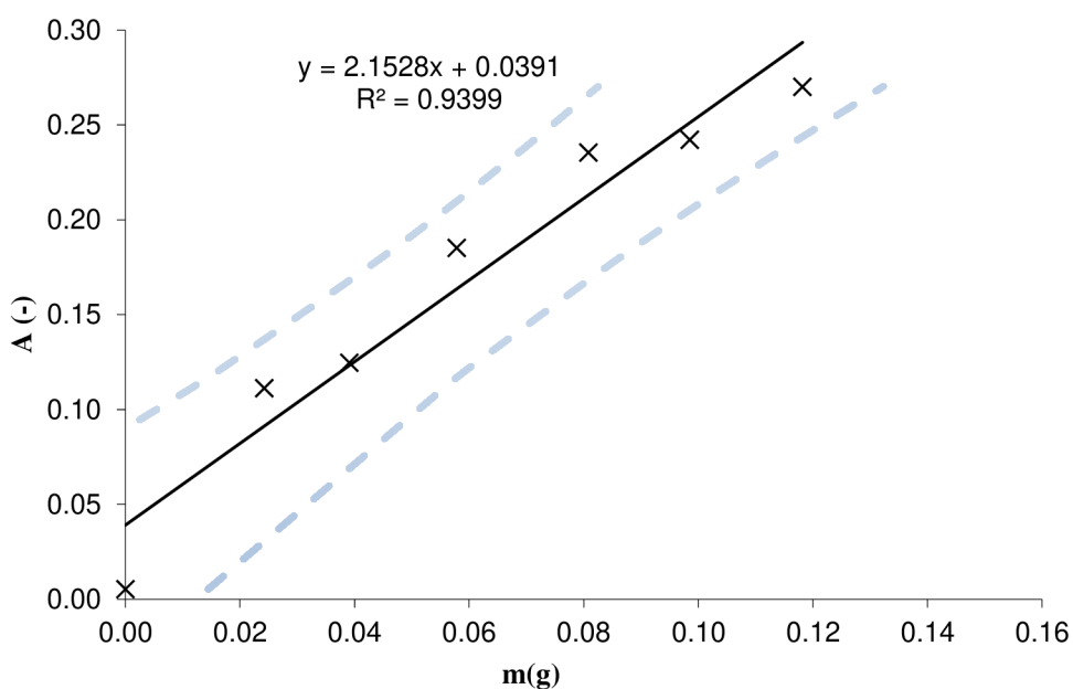
Graf 6: Kalibračná priamka závislosti absorbančie od hmotnosti plastu pre sériu M34+PHB a prvý pík
