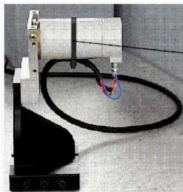
Obr. 4.4 Scintilační detektor
