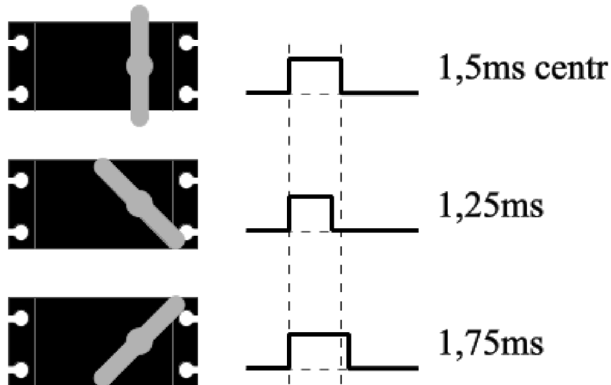
Obr. 5.5 Reakce serva na délku impulsu
