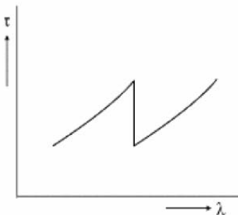
Obr. 2.3 Absorpční hrany
