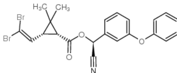
Obrázek č. 4: Strukturální vzorec deltamethrinu
