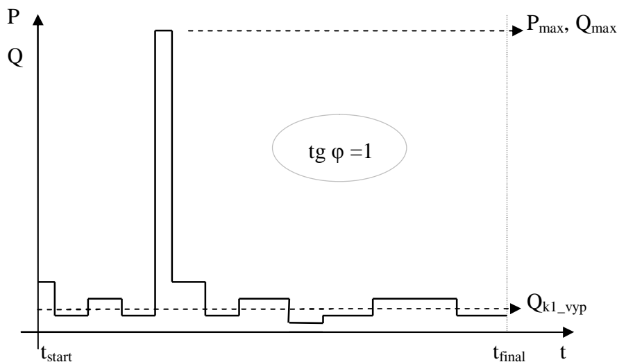
Obr. 9-1: Priebeh činného / jalového výkonu ( tg \varphi = 1 ) pre odmerané časové okno
