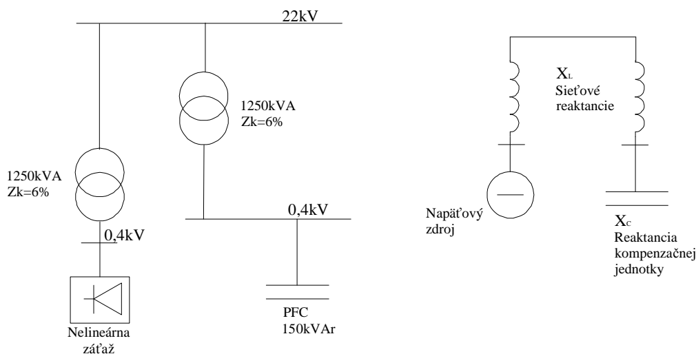
Obr. 6-14: Sieťová konfigurácia s pravdepodobnosťou sériovej rezonancie, ekvivalentný obvod.
