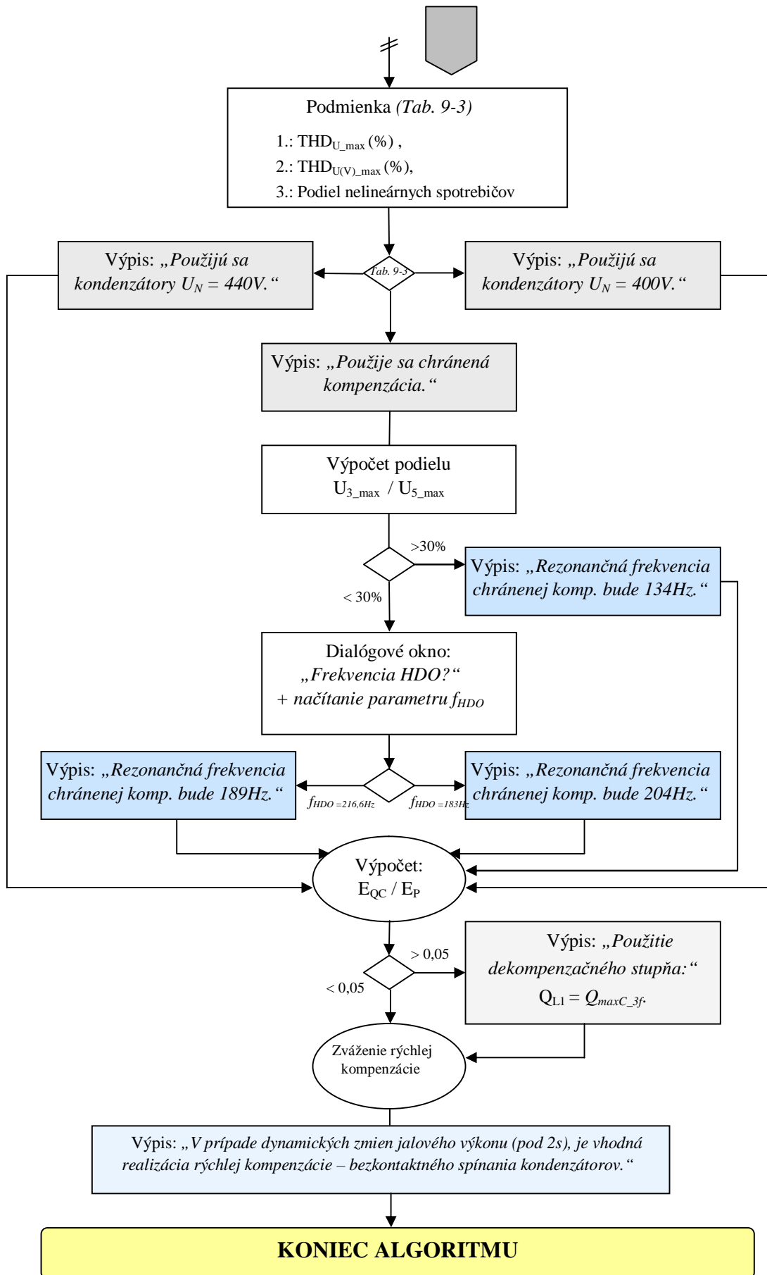
Obr. 9-3: Vývojový diagram ( 2 / 2 )
