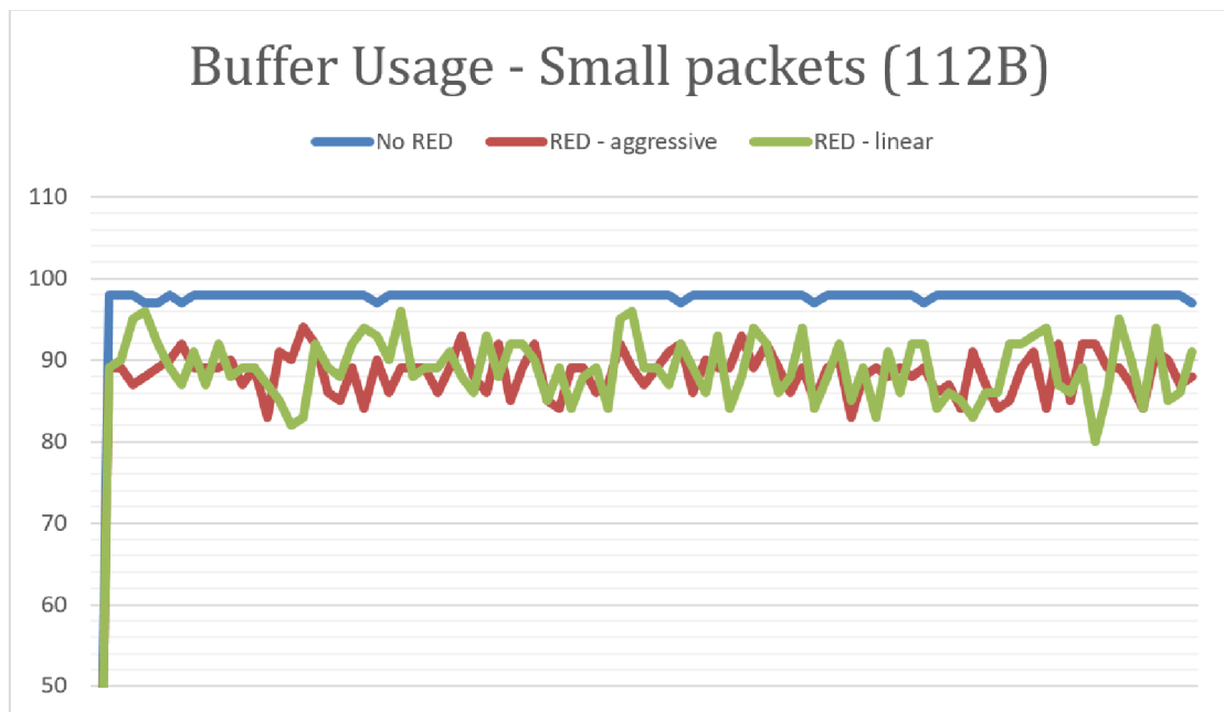
Obr. 6.2: Využitie fronty pri malých paketoch [11]
