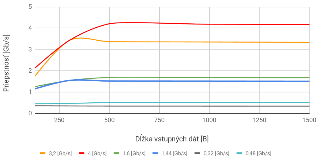
Obr. 5.4: Graf výsledkov testov 4, 5, 6 a 7
