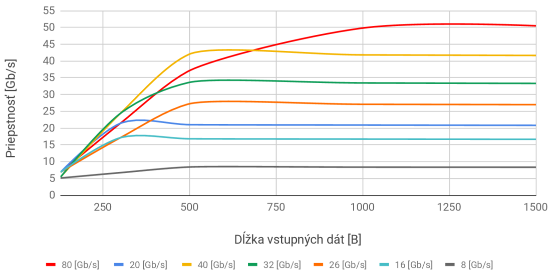
Obr. 5.3: Graf výsledkov testov 1, 2 a 3
