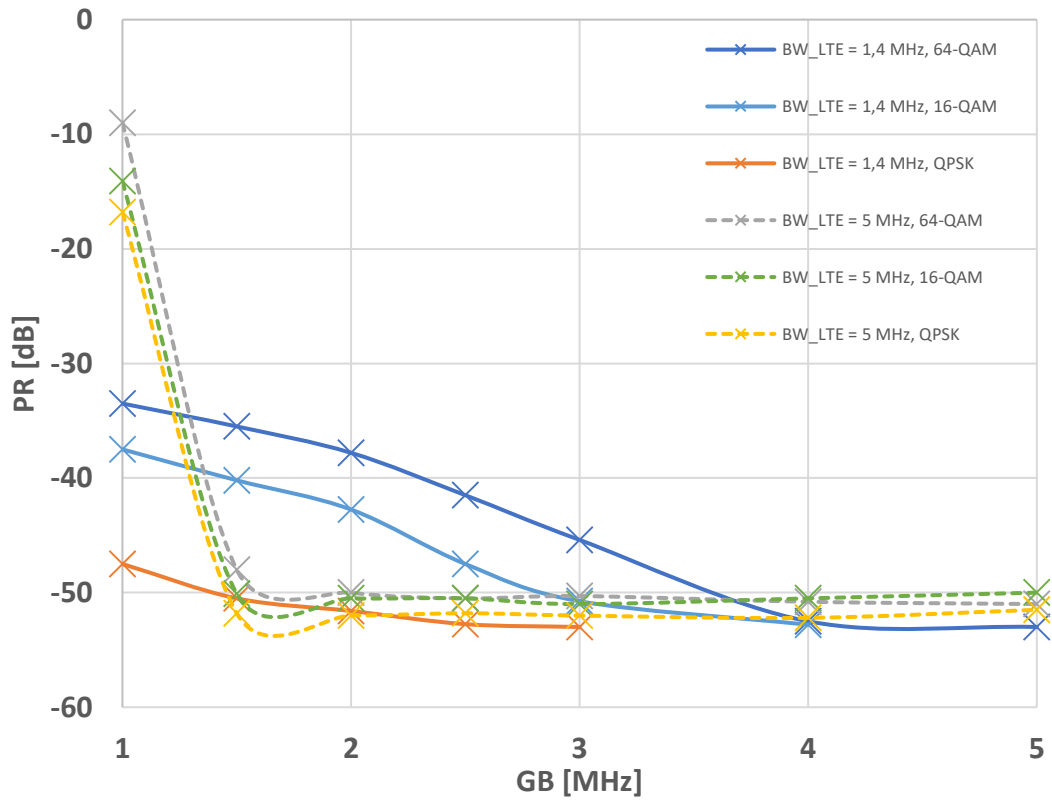
Obrázok 7-6: Závislosť PR na GB pre BW_{LTE} = 1,4 a 5 MHz, SF_{LoRa} = 10 , BW_{LoRa} = 500 kHz
