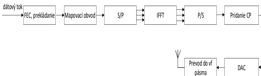
Obrázok 3-2: Blokóvá schéma LTE-DL
