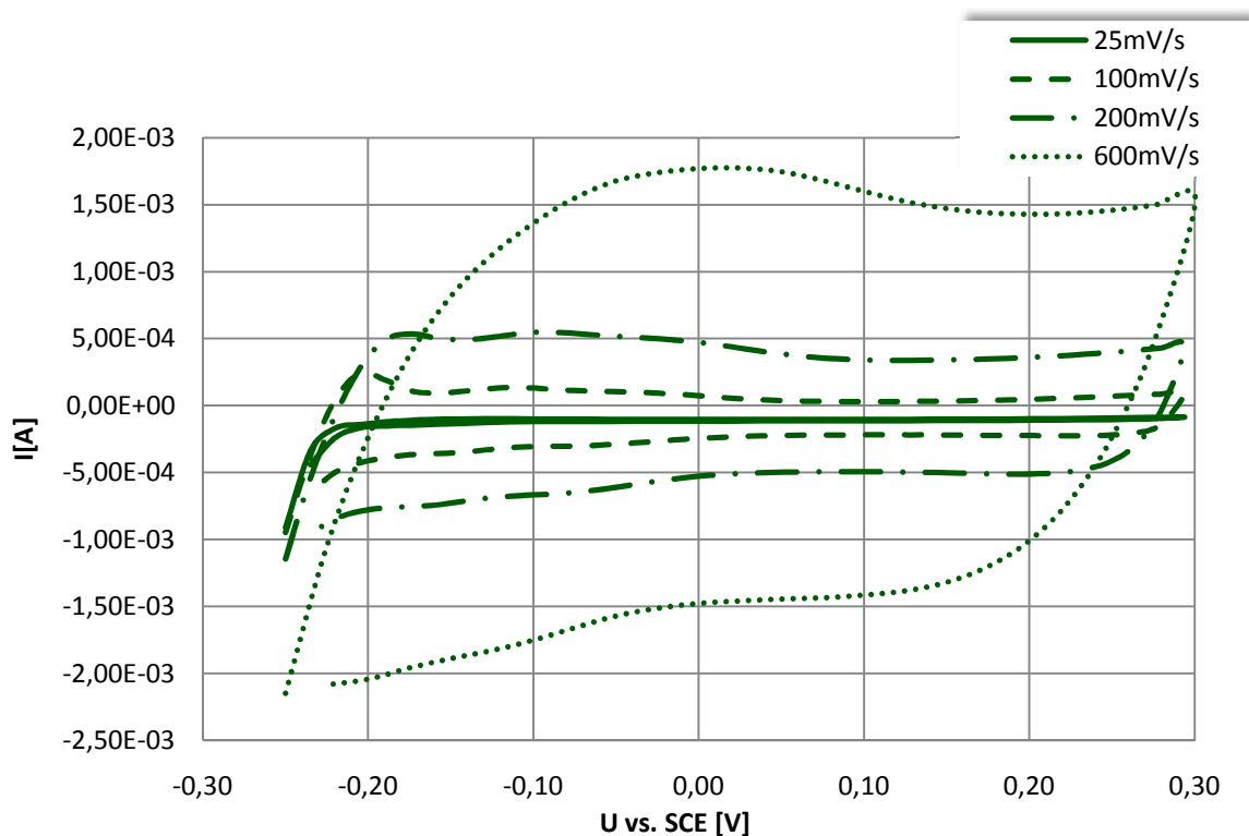
Obr. 3.11: A-V charakteristiky pro uhlík Vulcan XC-72 s 7 % Pt v závislosti na rychlostech změny potenciálu
