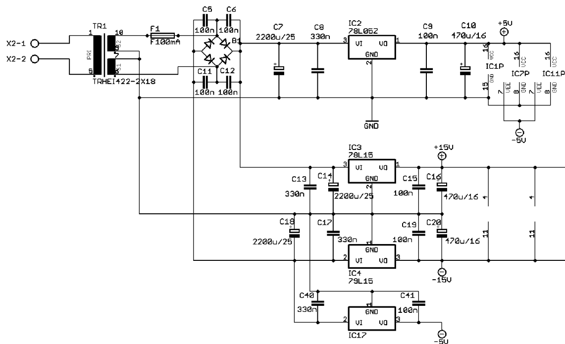
Obr. 5.2: Schéma zdroje
