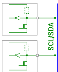
Obr. 1.5: Vnitřní struktura I 2 C rozhraní
